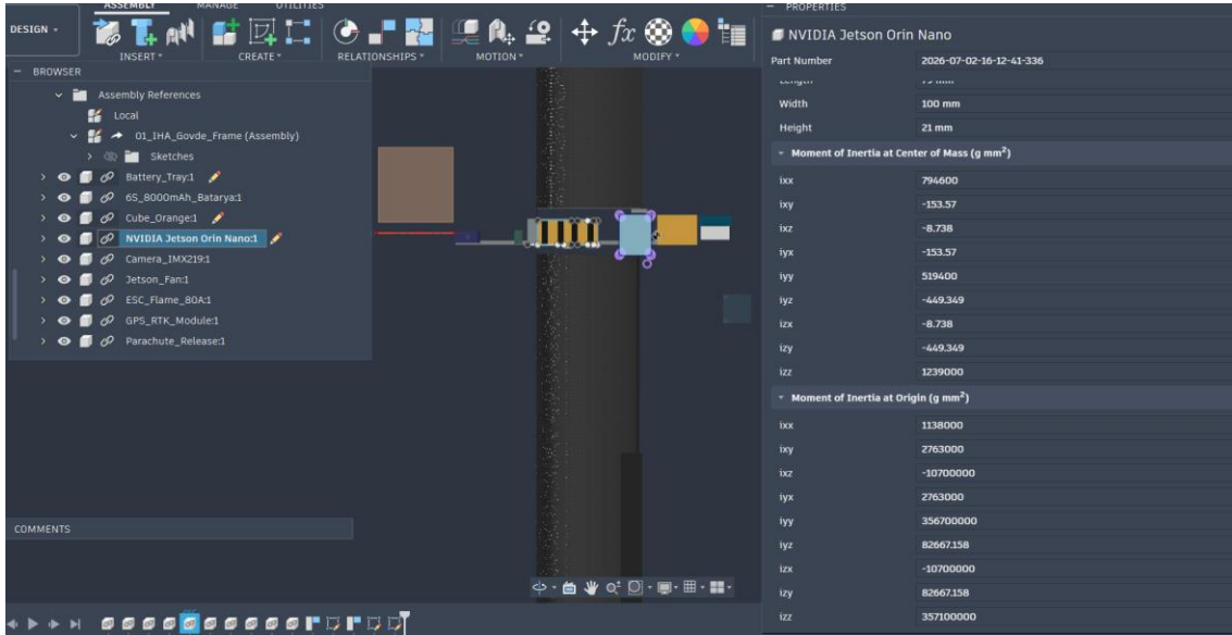
Şekil 3.1.2.25. Jetson'un ikinci CAD görünüşü. Güç, veri ve soğutma arayüzleri için montaj kontrolü gerekir.
