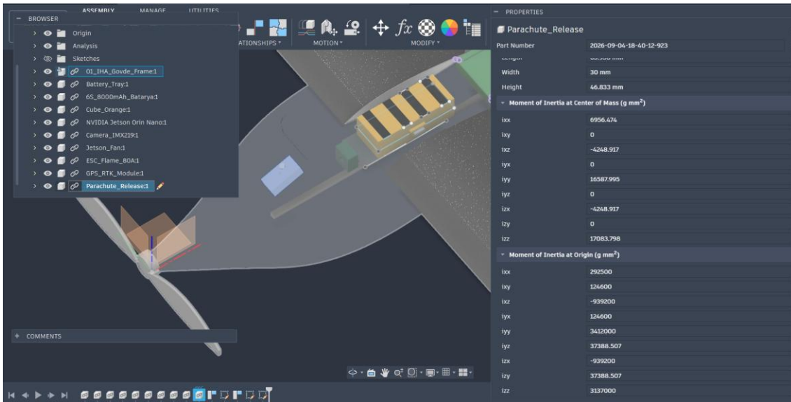
Şekil 3.1.2.31. Paraşüt bırakma mekanizmasının ikinci görünüşü. Tetikleme strokunun kapak ve gövde ile çakışmaması doğrulanmalıdır.
