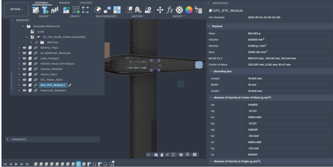
Şekil 3.1.2.22. GNSS/RTK modülünün RevC CAD yerleşimi.
