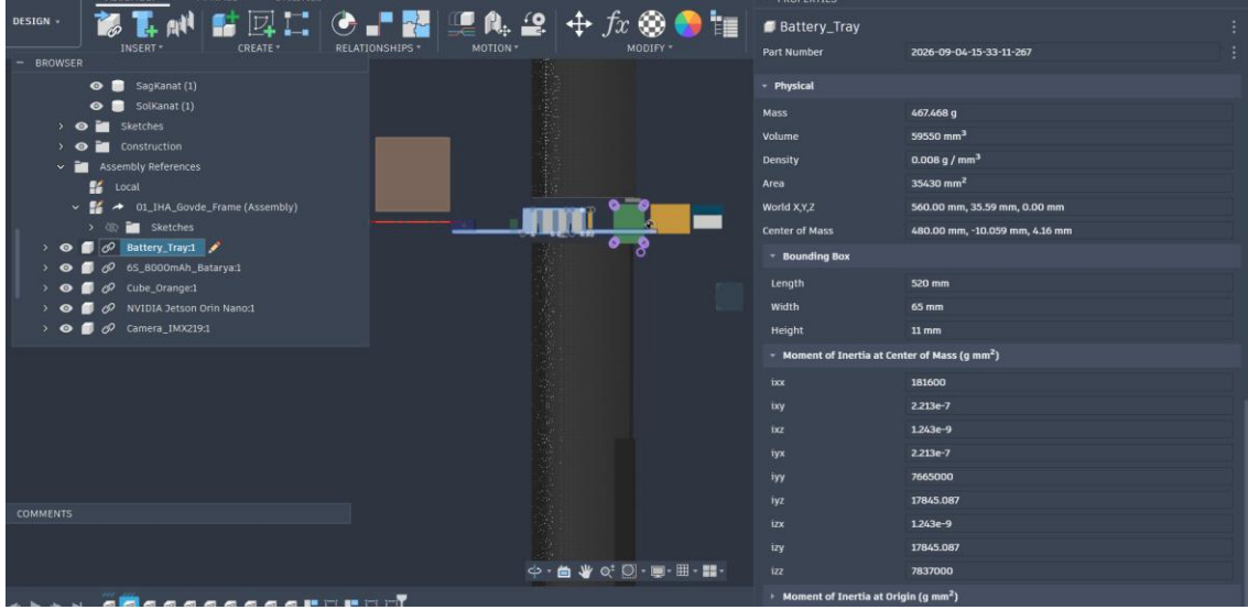
Şekil 3.1.2.16. Batarya tepsisinin gövde içi konumu ve batarya arayüzü.
