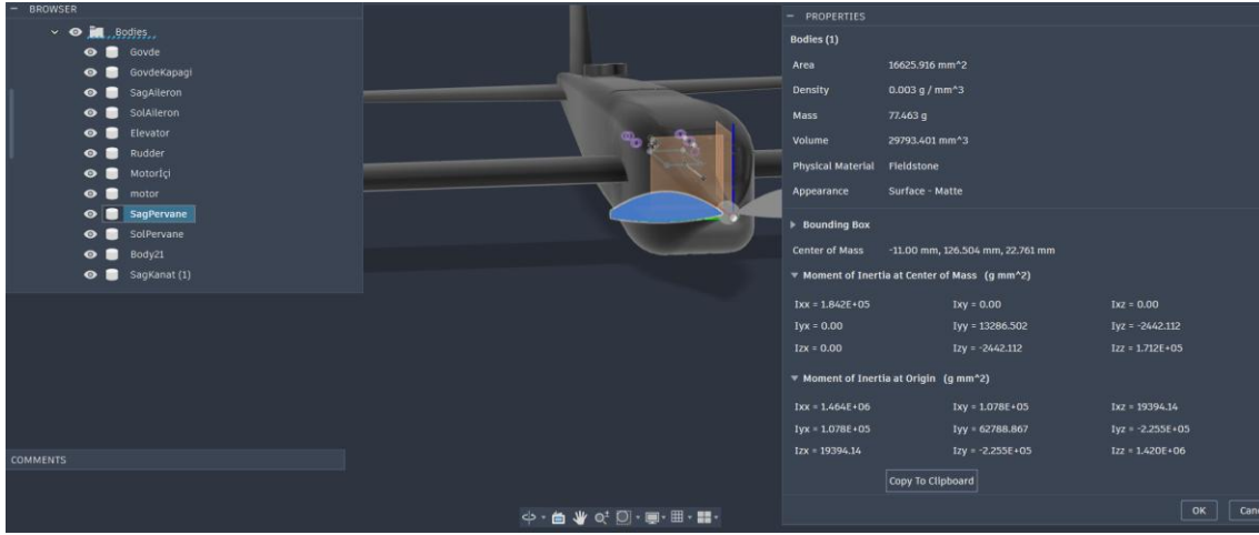
Şekil 3.1.2.12. Sağ pervanenin motor ve gövdeyle konum ilişkisi.
