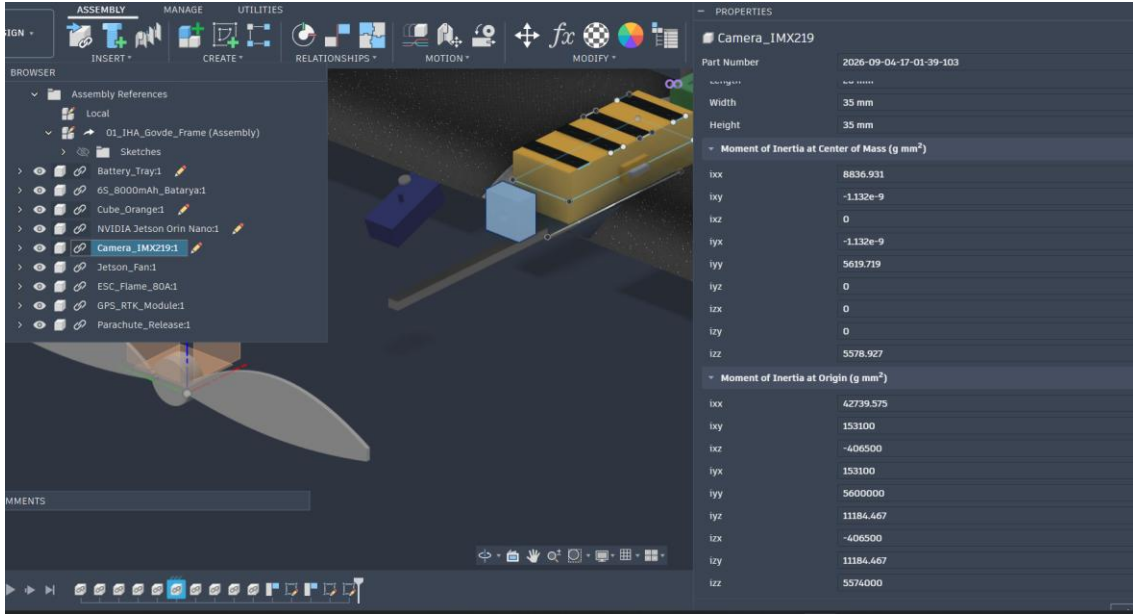
Şekil 3.1.2.29. Kameranın ikinci görünüşü. Görüş eksen ve gövde açıklığı hizası üretim sonrası kontrol edilmelidir.
