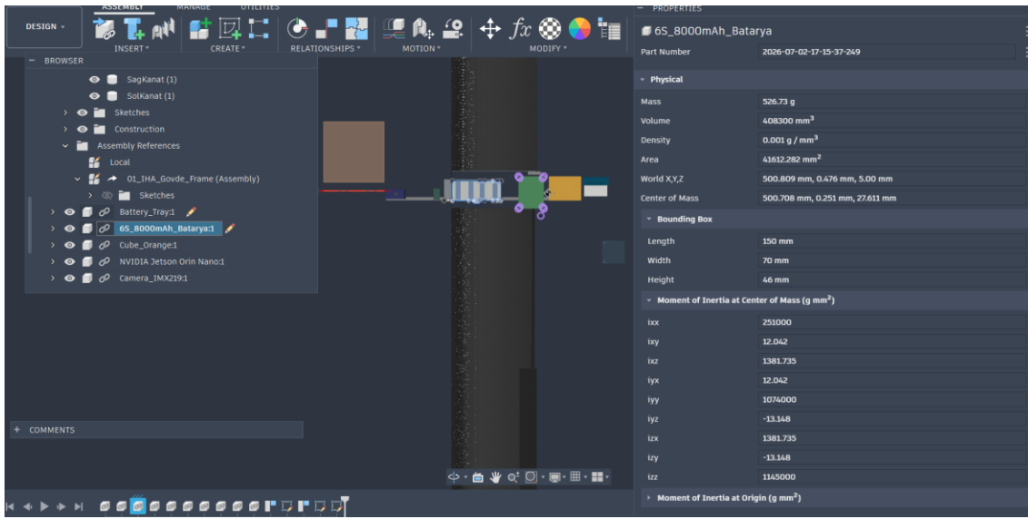
Şekil 3.1.2.14. 6S 8000 mAh bataryanın boyutları, kütle özelliği ve gövde içindeki konumu.
