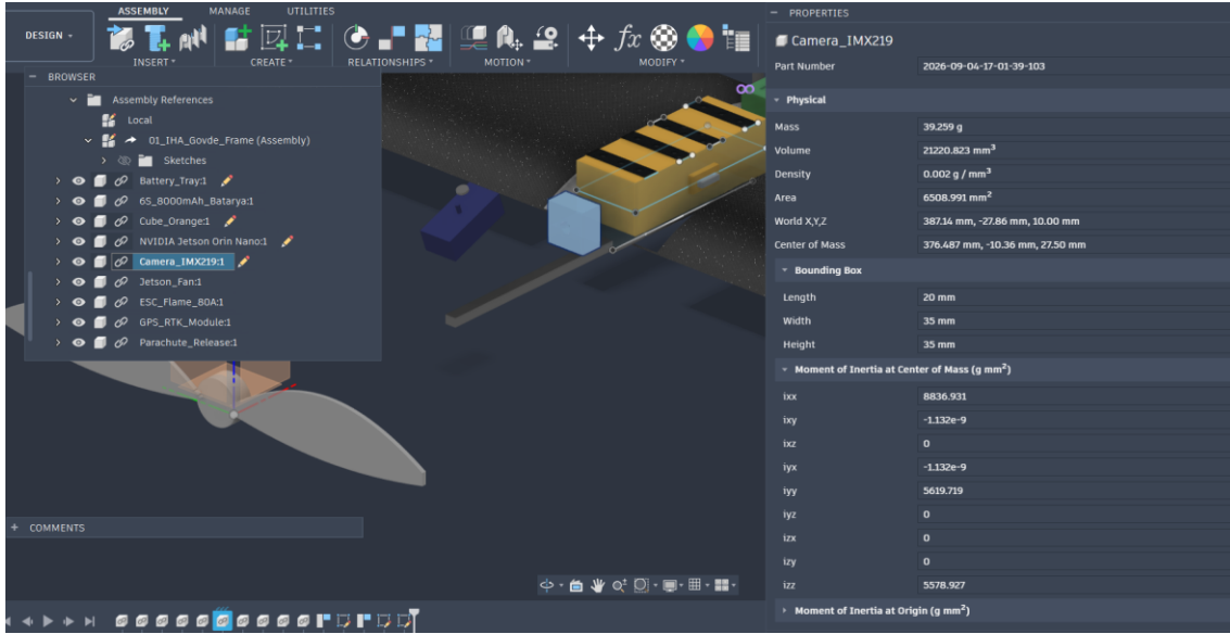
Şekil 3.1.2.28. IMX219 sınıfı kameranın gövde içi/önü yerleşim görünüşü.
