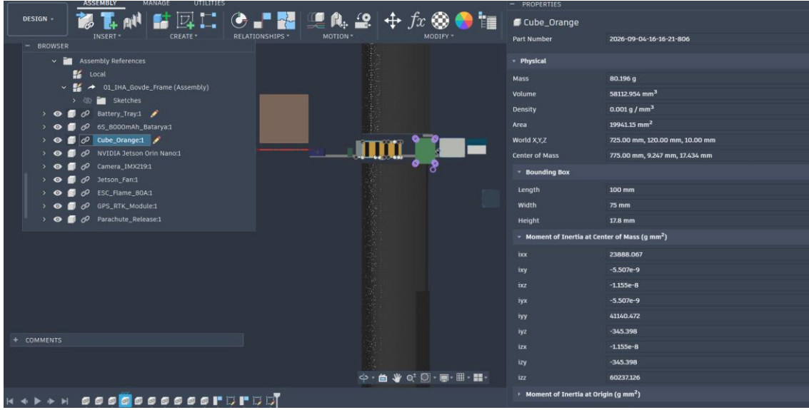
Şekil 3.1.2.20. Cube Orange uçuş kontrol kartının CAD zarfı, kütlesi ve yerleşimi.
