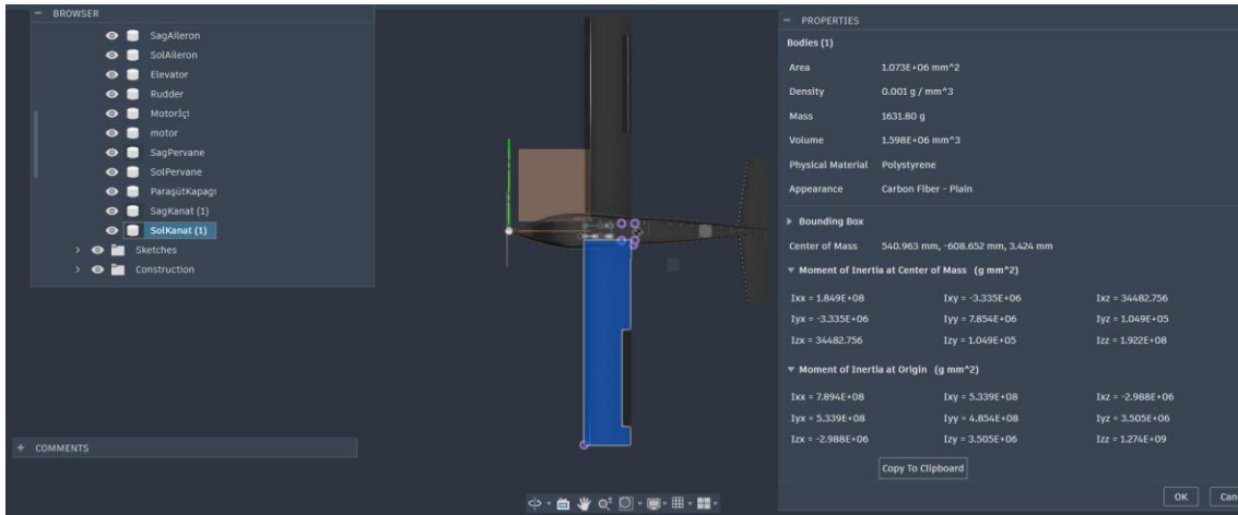
Şekil 3.1.2.3. Sol kanadın RevC montaj yerleşimi. Sağ-sol geometrik eşleşme ayrı bir montaj kontrol maddesidir.
