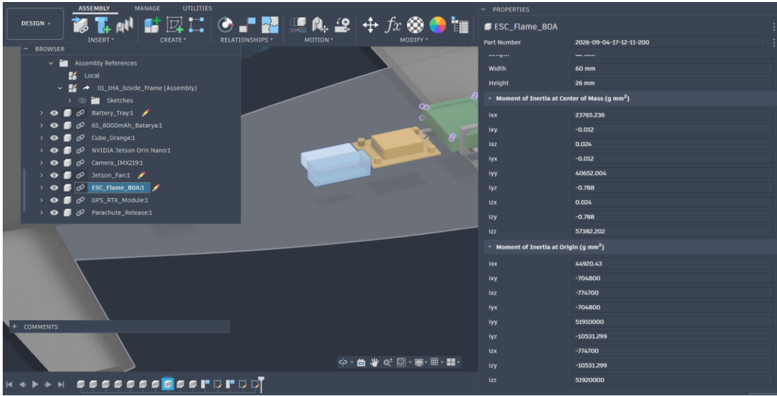
Şekil 3.1.2.19. ESC yerleşiminin ikinci görünüşü. Kablo çıkışları ve termal erişim montajda kontrol edilmelidir.
