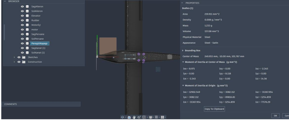
Şekil 3.1.2.32. Paraşüt kapağının gövde üzerindeki konumu ve kurtarma sistemi erişim arayüzü.
