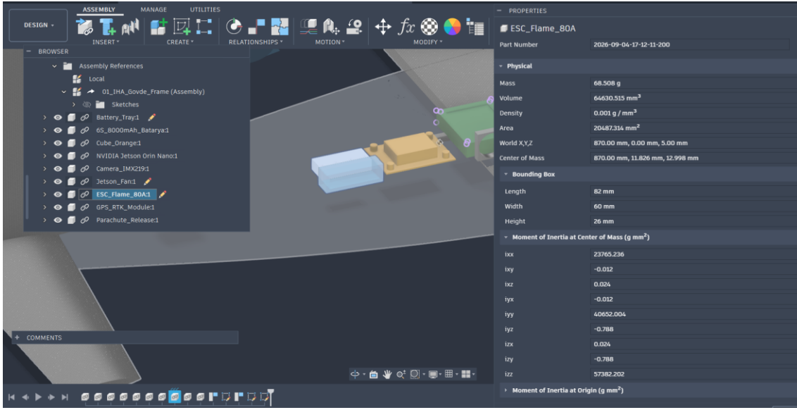
Şekil 3.1.2.18. ESC'nin gövde içi konumu ve çevre bileşenlerle mesafesi.
