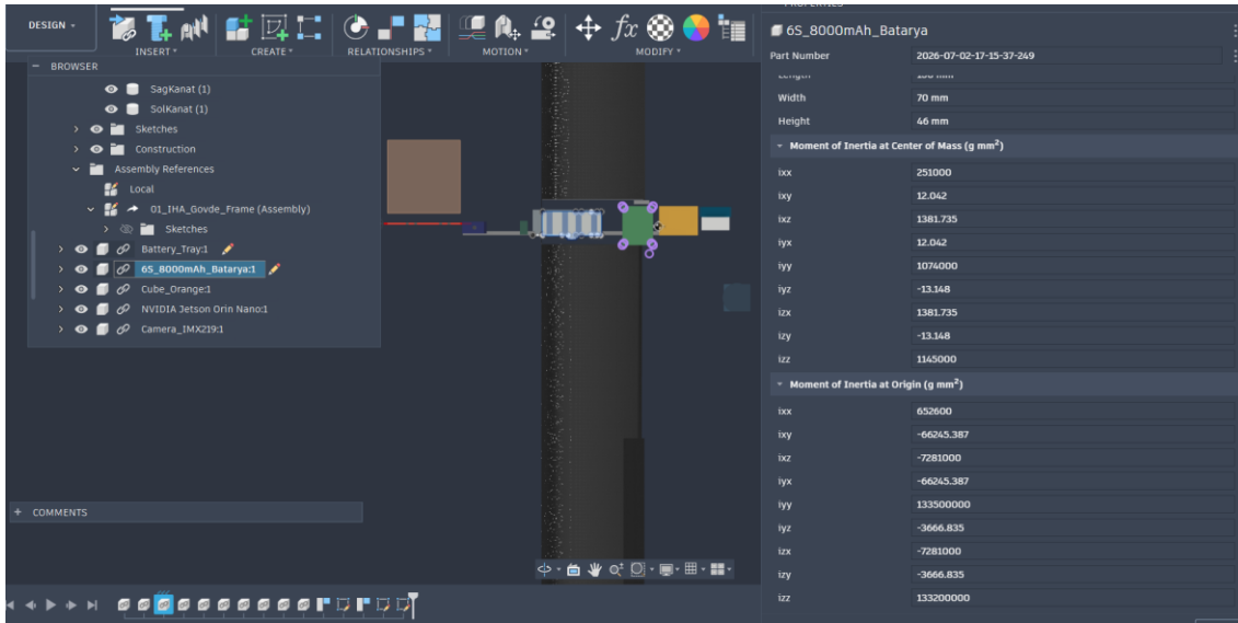
Şekil 3.1.2.15. Batarya yerleşiminin ikinci CAD görünüşü. Çıkarılabilirlik ve konektör erişimi montaj kontrolünde doğrulanmalıdır.
