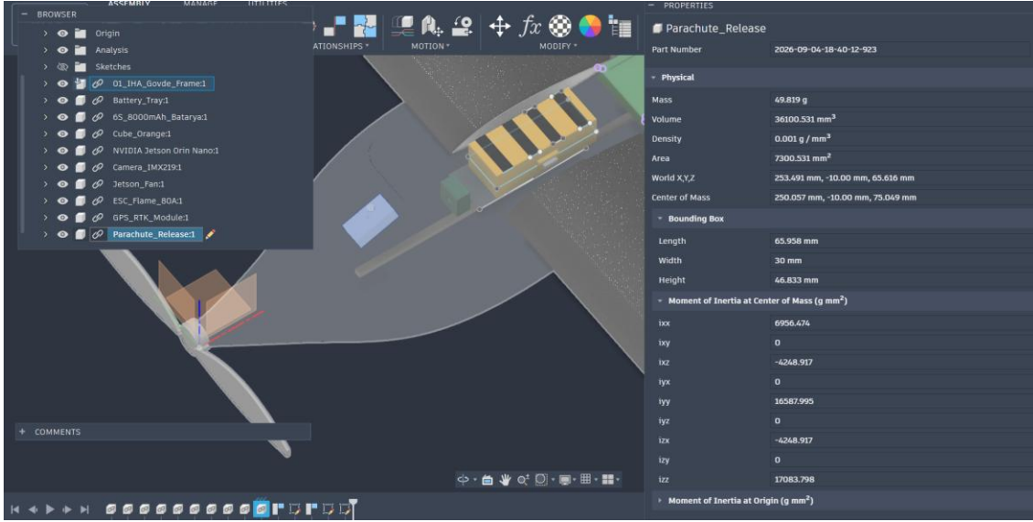
Şekil 3.1.2.30. Paraşüt bırakma mekanizmasının FDR CAD zarfı, kütlesi ve gövde içi konumu.
