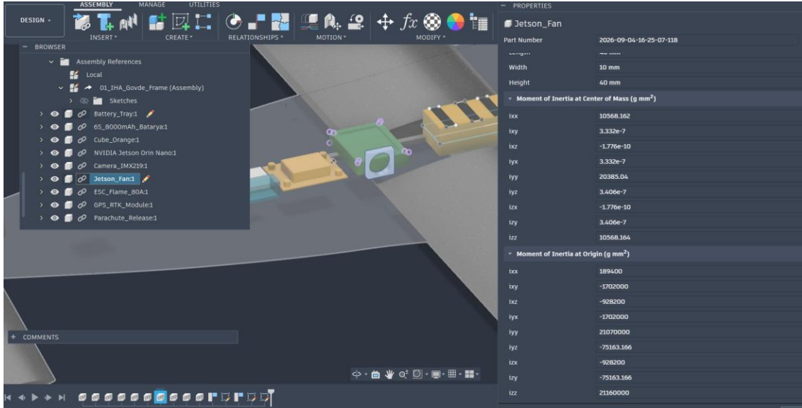
Şekil 3.1.2.27. Fan yerleşiminin ikinci görünüşü. Fan akışının gövde çıkışlarıyla sürekliliği üretim sonrasında doğrulanmalıdır.
