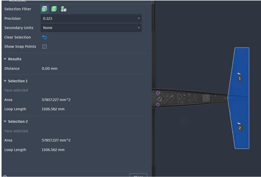
Şekil 3.1.2.5. RevC yatay kuyruk planformunda iki simetrik seçili yüz için CAD Measure sonucu (her bir yüz: 57.857,227 mm 2 ).
