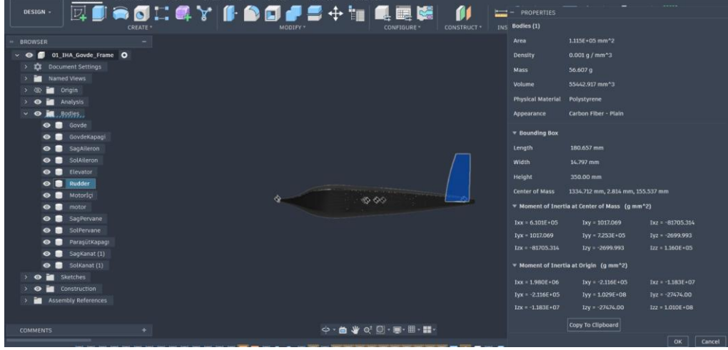
Şekil 3.1.2.9. Rudder CAD Properties kaydında merkez koordinatı X=1.334,712 mm olarak görülmektedir.
