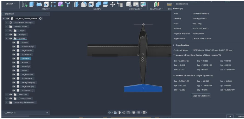
Şekil 3.1.2.7. Elevatör CAD Properties kaydında merkez koordinatı X=1.375,380 mm olarak görülmektedir.
