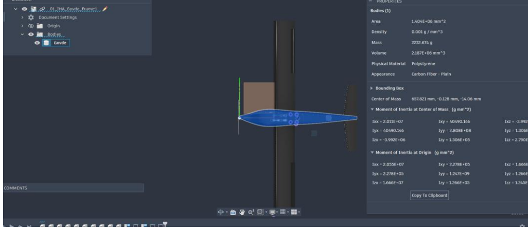
řekil 3.1.2.4. Gvde ana erevesi ve kanat-kuyruk-alt sistem yerleşim ilişkisi.
