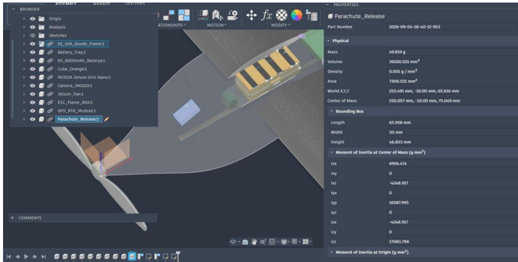
Şekil 3.1.2.10. Paraşüt bırakma mekanizmasının FDR CAD zarfı, kütlesi ve gövde içi konumu.
