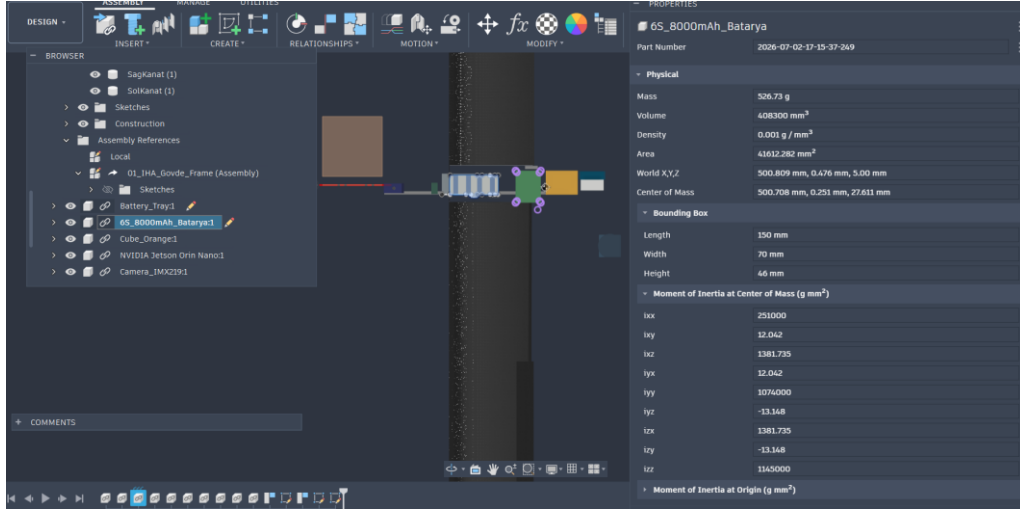
Şekil 3.1.2.9. 6S 8000 mAh bataryanın boyutları, kütle özelliği ve gövde içindeki konumu.
