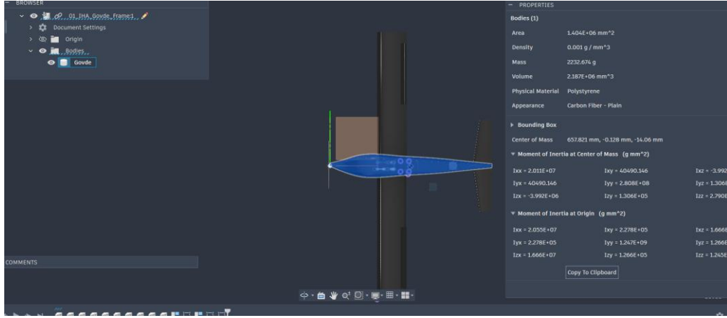
Şekil 3.1.2.4. Gövde ana çerçevesi ve kanat-kuyruk-alt sistem yerleşim ilişkisi.
