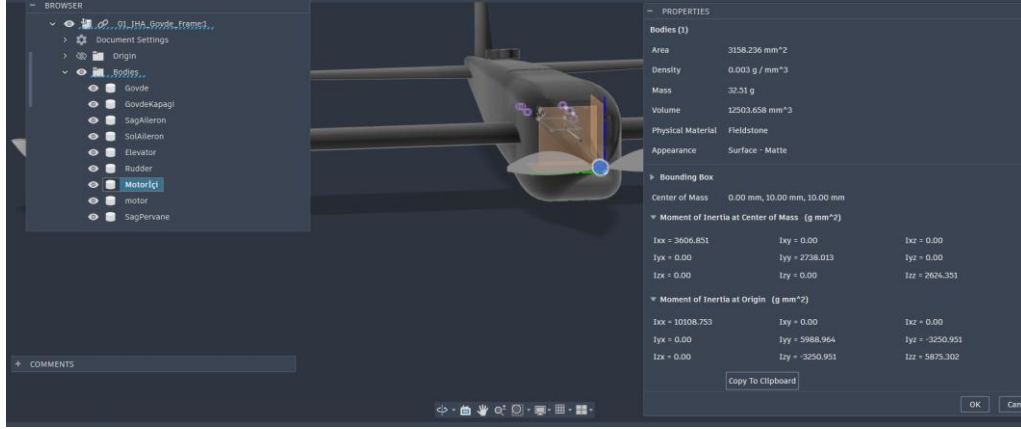
Şekil 3.1.2.8. Motorun gövde içi yerleşimi. Kablo ve taşıyıcı arayüzler montaj doğrulamasında ayrıca kontrol edilmelidir.
