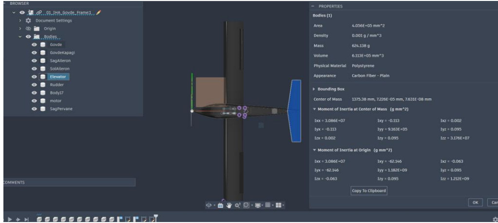
Şekil 3.1.2.7. Elevator ve T-kuyruk bağlantısı. Görsel, arka gövde ile hareketli yatay yüzeyin konum ilişkisini gösterir.
