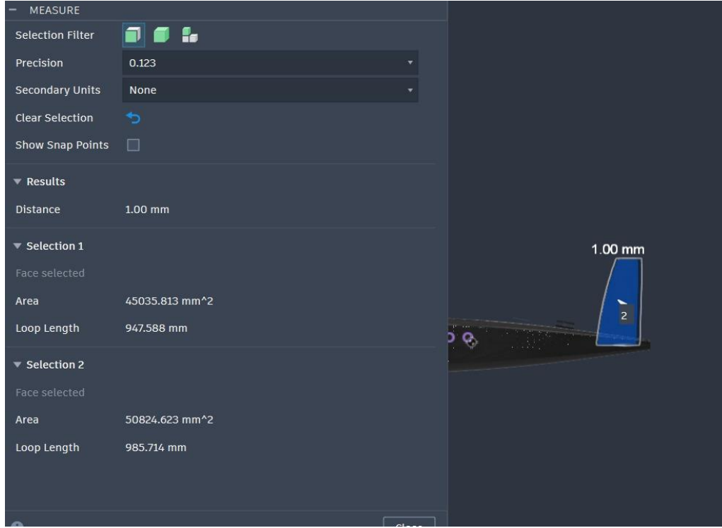
Şekil 3.1.2.6. RevC dikey kuyrukta seçili iki planform yüzünün CAD Measure sonuçları (45.035,813 mm 2 ve 50.824,623 mm 2 ).
