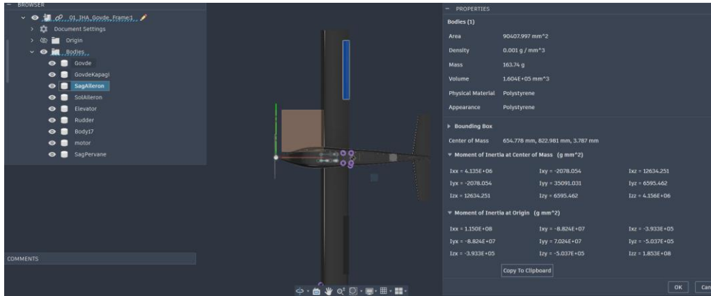
Şekil 3.1.2.4. Sağ aileronun kanat firar kenarındaki yerleşimi ve parça özellikleri.
