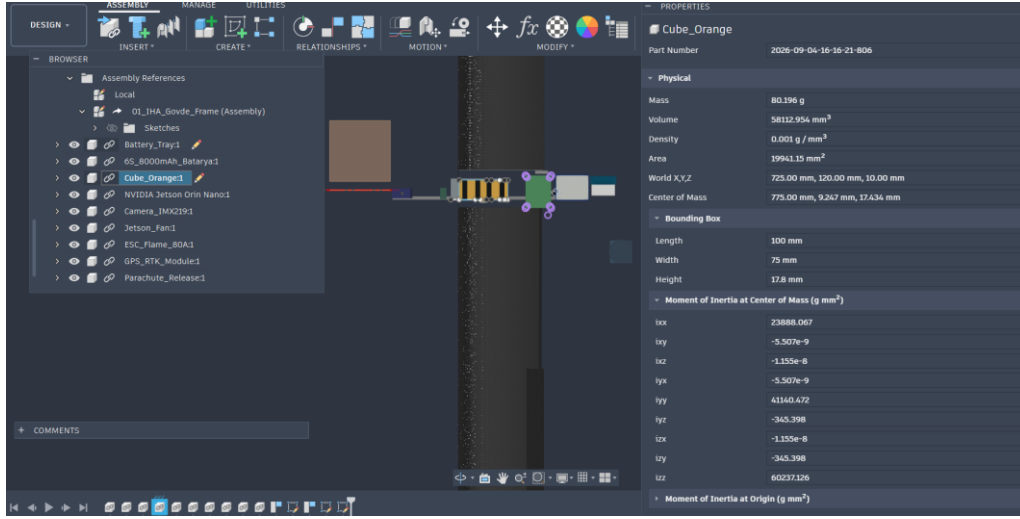
Şekil 3.1.2.15. Cube Orange uçuş kontrol kartının CAD zarfı, kütlesi ve yerleşimi.
