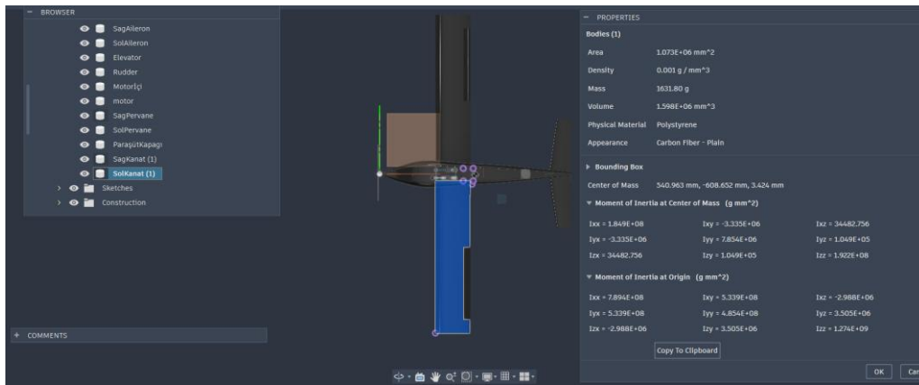
Şekil 3.1.2.3. Sol kanadın RevC montaj yerleşimi. Sağ-sol geometrik eşleşme ayrı bir montaj kontrol maddesidir.
