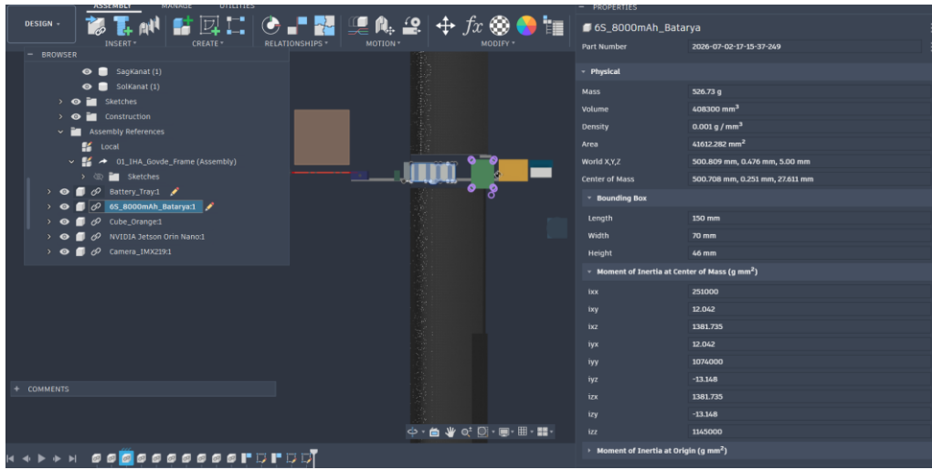
Şekil 3.1.2.12. 6S 8000 mAh bataryanın boyutları, kütle özelliği ve gövde içindeki konumu.
