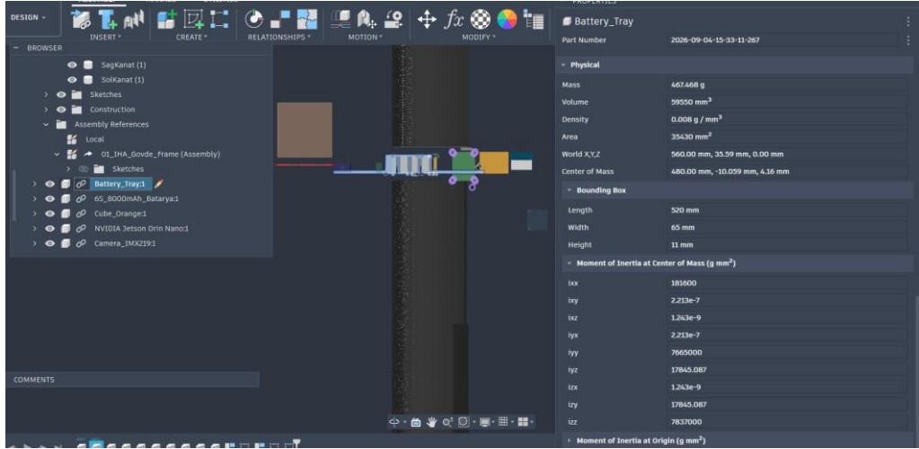
Şekil 3.1.2.13. Batarya tepsisinin gövde içi konumu ve batarya arayüzü.
