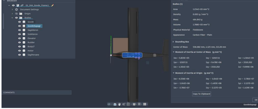
Şekil 3.1.2.7. Gövde kapağının RevC montajındaki konumu ve bakım erişim bölgesi.
