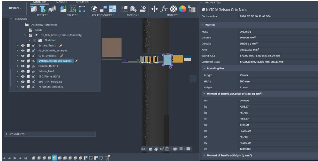
Şekil 3.1.2.17. NVIDIA Jetson Orin Nano'nun CAD kütle ve zarf bilgileriyle gövde içi yerleşimi.
