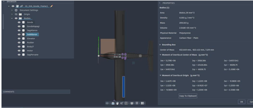
Şekil 3.1.2.5. Sol aileronun RevC yerleşimi. Sağ-sol hareketli yüzeylerin birbirine çarpma ve sapma zarfı kontrol edilmelidir.
