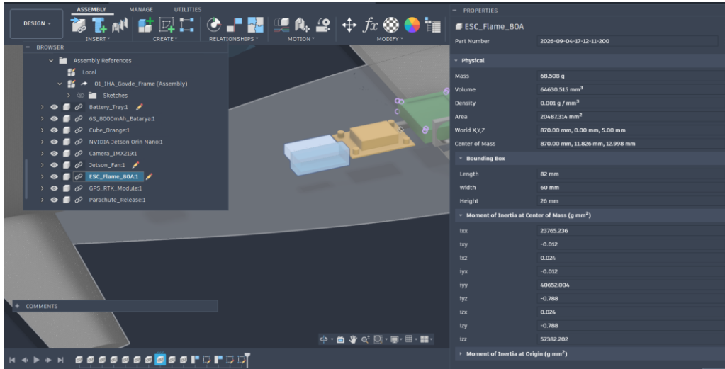
Şekil 3.1.2.14. ESC'nin gövde içi konumu ve çevre bileşenlerle mesafesi.
