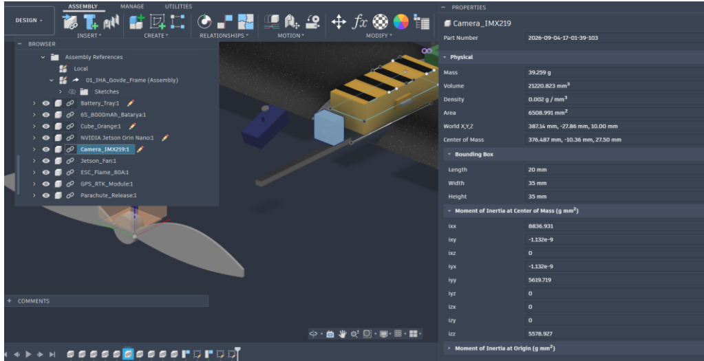
Şekil 3.1.2.19. IMX219 sınıfı kameranın gövde içi/önü yerleşim görünüşü.
