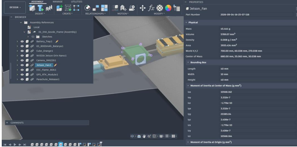
Şekil 3.1.2.18. Jetson fanı ve görev bilgisayarı çevresindeki soğutma zarfı.
