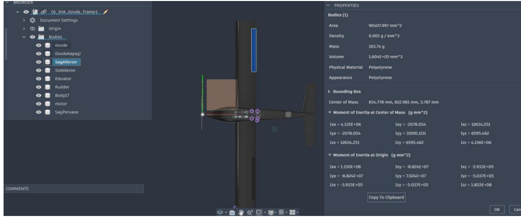
Şekil 3.1.2.4. Sağ aileronun kanat firar kenarındaki yerleşimi ve parça özellikleri.
