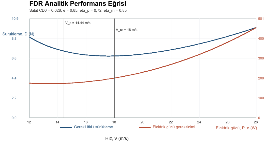
Şekil 3.1.6.4. FDR geometri-kütle girdileriyle gerekli sürüklenme ve elektrik gücü eğrisi. Eğri, sabit C_{D0} , e , \eta_p ve \eta_m varsayımlarına dayanır.
