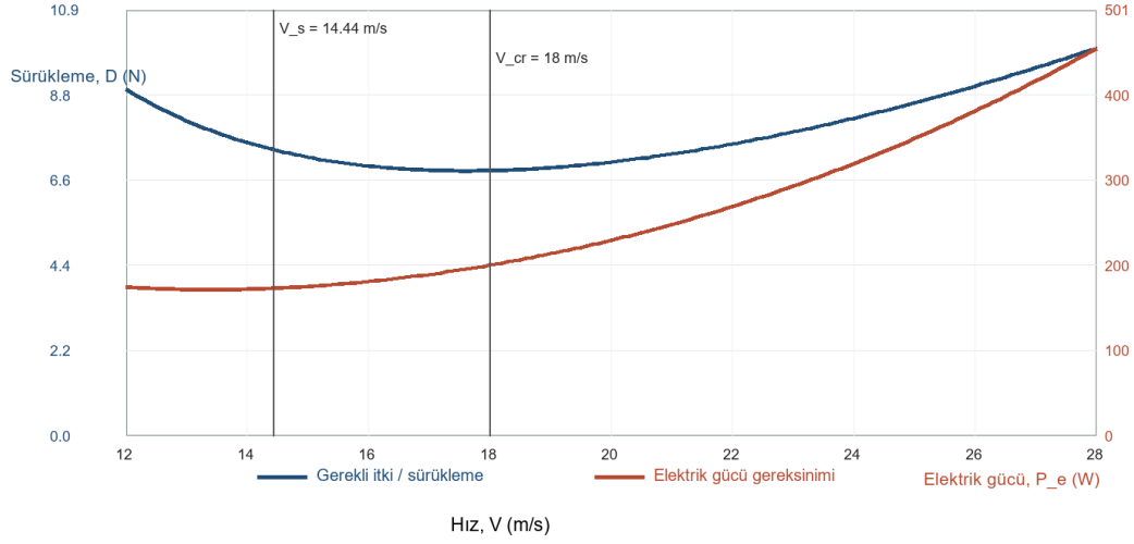
Şekil 3.1.6.4. FDR geometri-kütle girdileriyle gerekli sürüklenme ve elektrik gücü eğrisi. Eğri, sabit C_D0, e, eta_p ve eta_m varsayımlarına dayanır.
