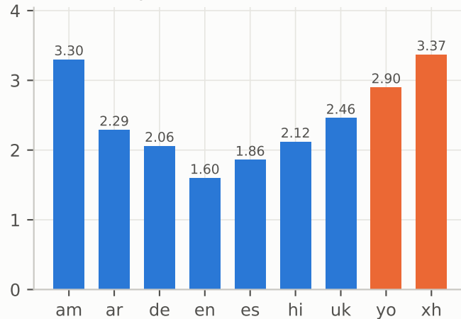
mT5 fertility (subwords / word)
