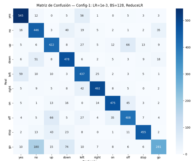
Fig. 8: Matriz de confusión del mejor Modelo A (Configuración 1) sobre los datos de prueba.
