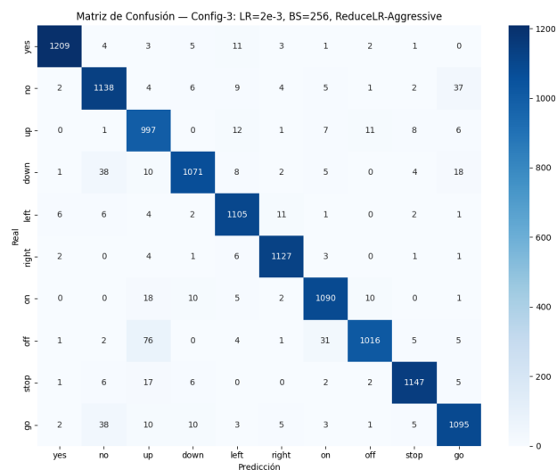
Fig. 20: Matriz de confusión del Modelo B aumentado sobre el conjunto de prueba.
