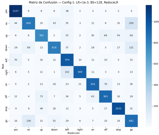
Fig. 12: Matriz de confusión del Modelo A aumentado sobre el conjunto de prueba.
