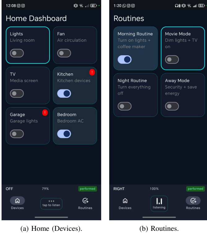
Fig. 21: Aplicación Android: demo de la interfaz para dispositivos y rutinas.
