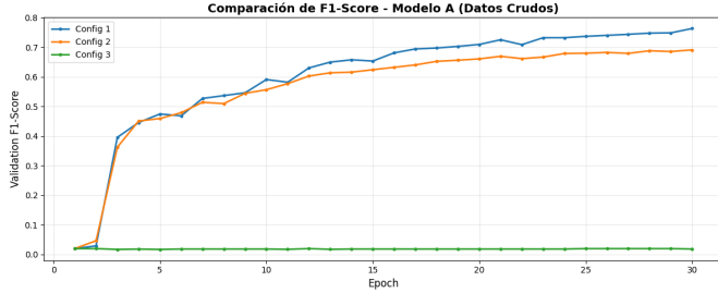
Fig. 6: Evolución del F1-Score macro en validación para el mejor Modelo A (Configuración 1).
