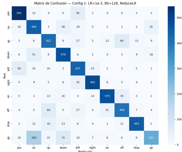
Fig. 7: Matriz de confusión del mejor Modelo A (Configuración 1) sobre los datos de prueba.
