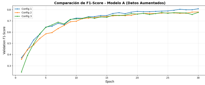
Fig. 10: Evolución del F1-Score macro para el mejor Modelo A aumentado.
