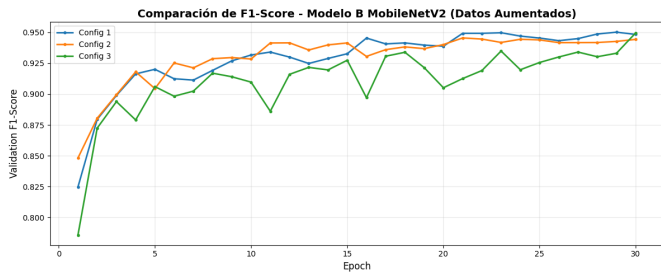
Fig. 17. Evolución del F1-Score macro para el mejor Modelo B aumentado.
