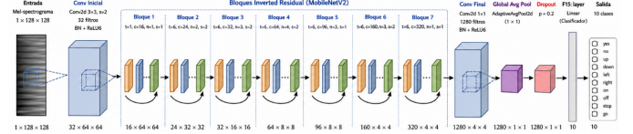
Fig. 2. Diagrama visual de la arquitectura del Modelo B.
