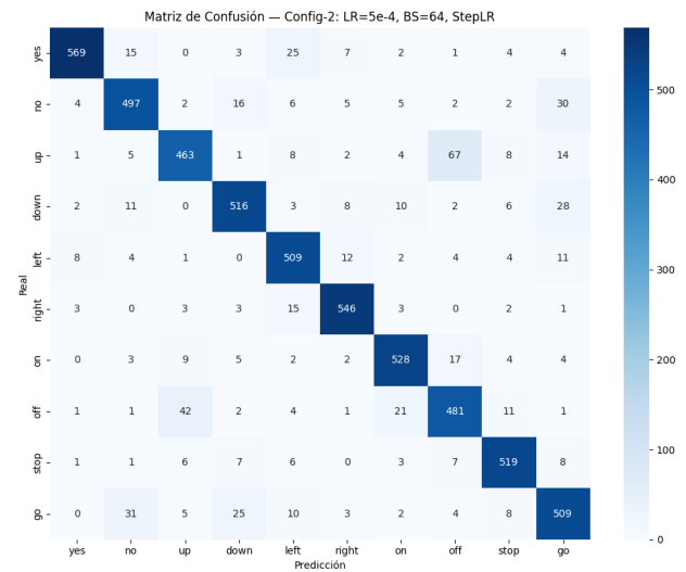
Fig. 6. Matriz de confusión del mejor Modelo A (Configuración 2) sobre los datos de prueba.
