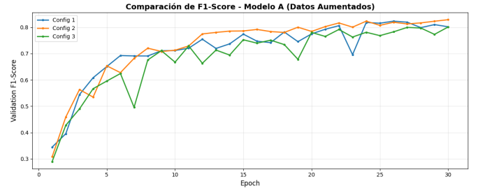
Fig. 9. Evolución del F1-Score macro para el mejor Modelo A aumentado.
