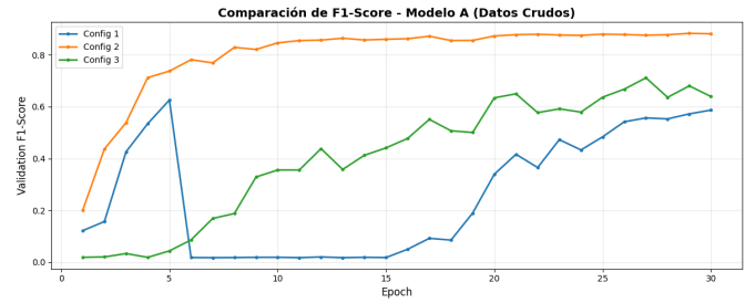
Fig. 5. Evolución del F1-Score macro en validación para el mejor Modelo A (Configuración 2).
