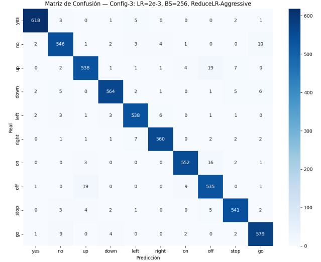
Fig. 14. Matriz de confusión del Modelo B (datos crudos) sobre el conjunto de prueba.
