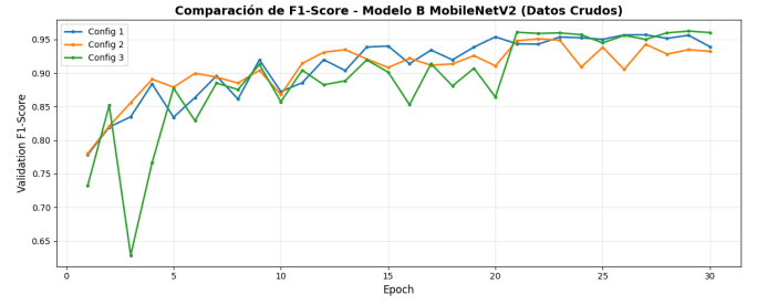
Fig. 13. Evolución del F1-Score macro para el mejor Modelo B (datos crudos).
