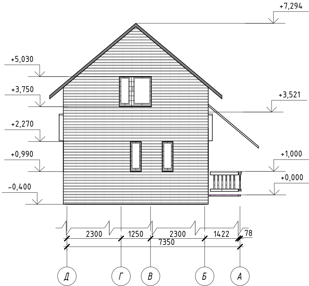
Западный 1 : 100
