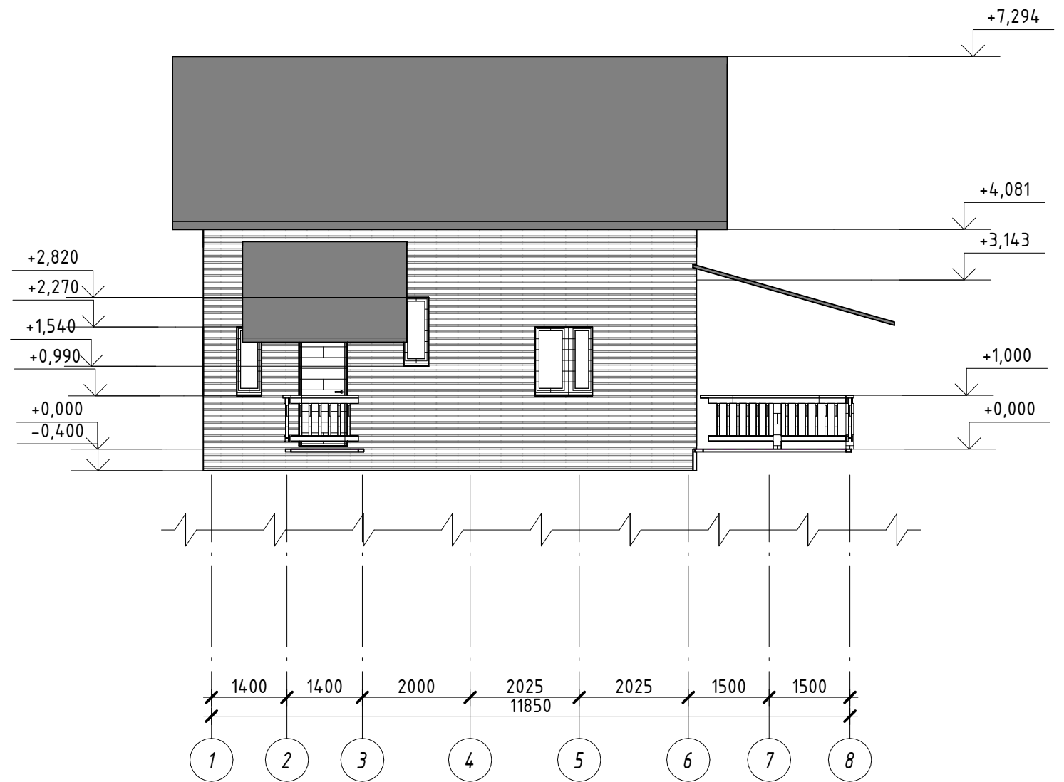
Южный 1 : 100
