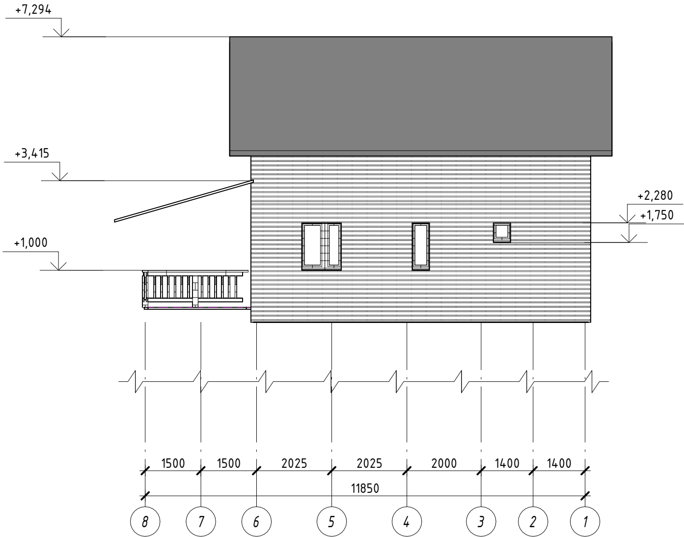
Северный 1 : 100
