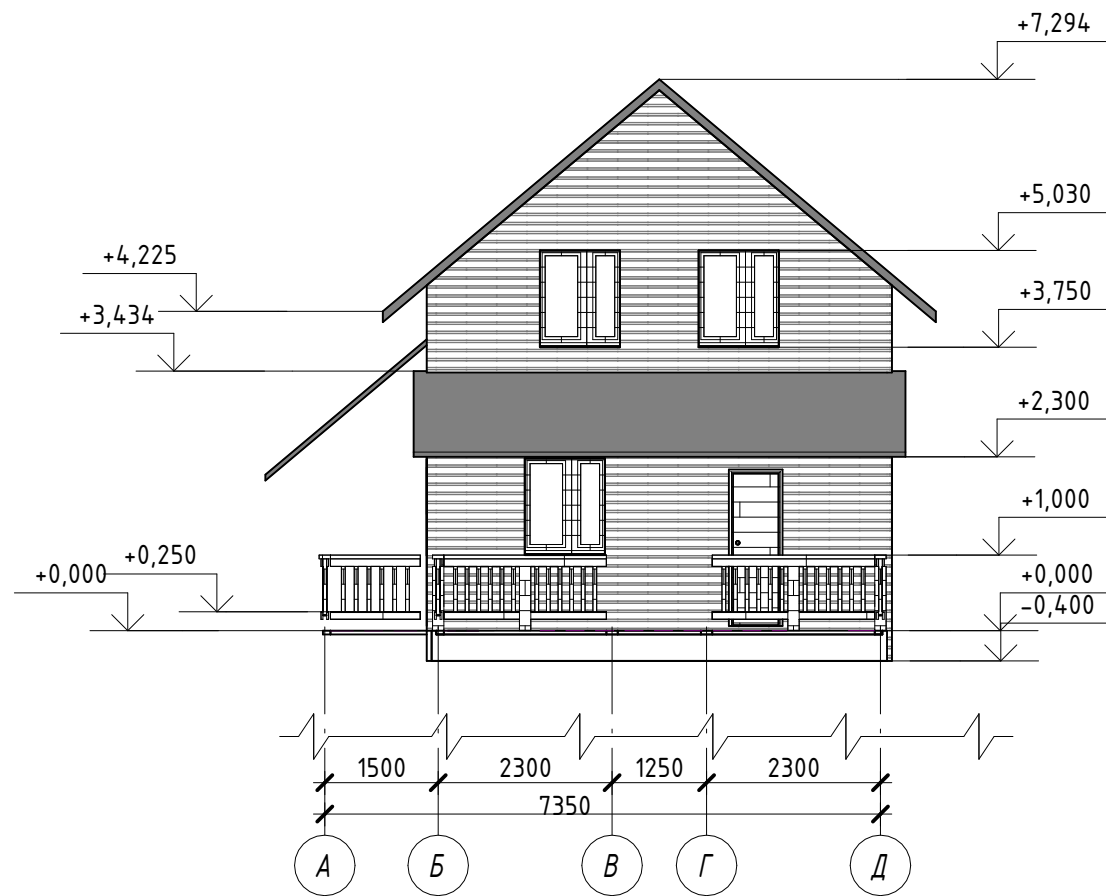
Восточный 1 : 100
