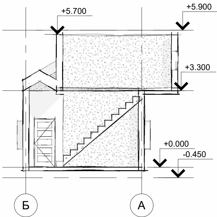
Сечение 3-3 1:100
