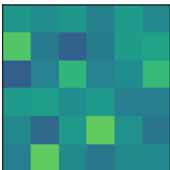
Pair (0,5)
