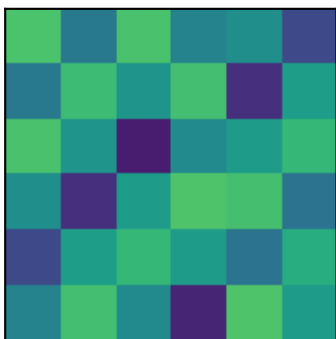
Pair (0,1)
