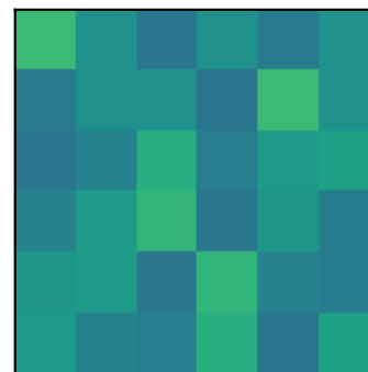
Pair (0,4)
