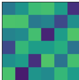
Pair (0,3)
