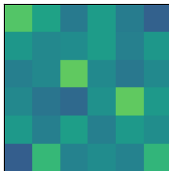
Pair (0,2)
