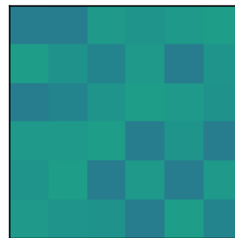
Pair (2,5)
