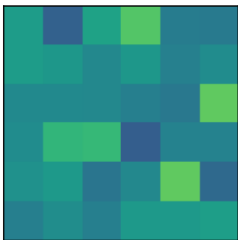
Pair (1,5)
