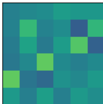
Pair (3,5)
