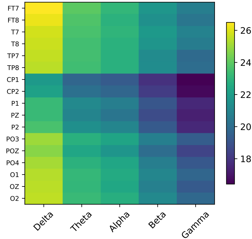
Alert (DE)
