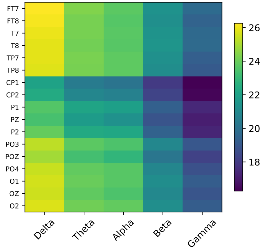
Drowsy (DE)
