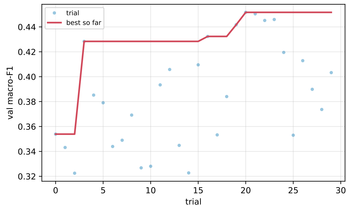
MLP
