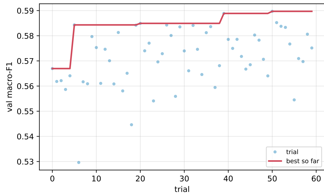
MLP
