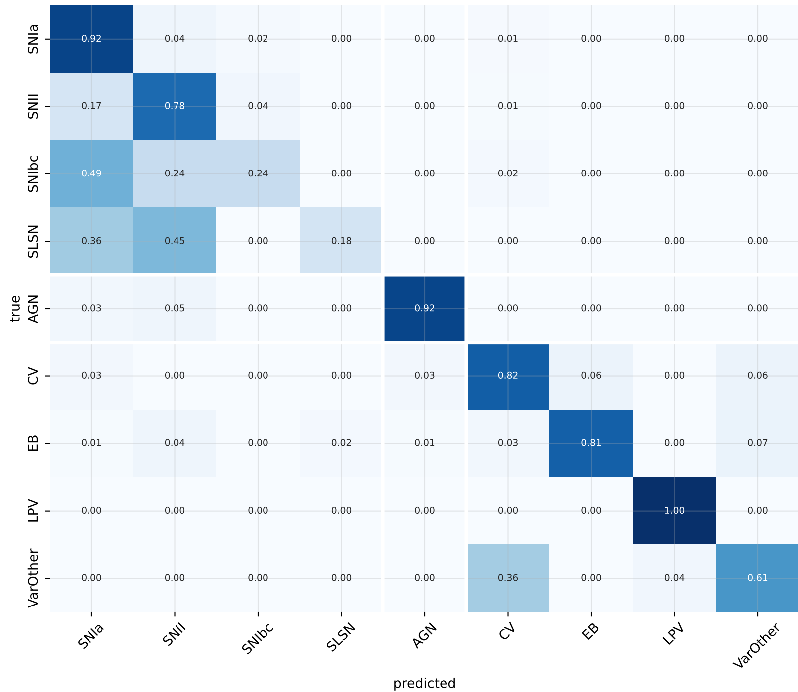
Hierarchical XGBoost (macro-F1 0.706)
