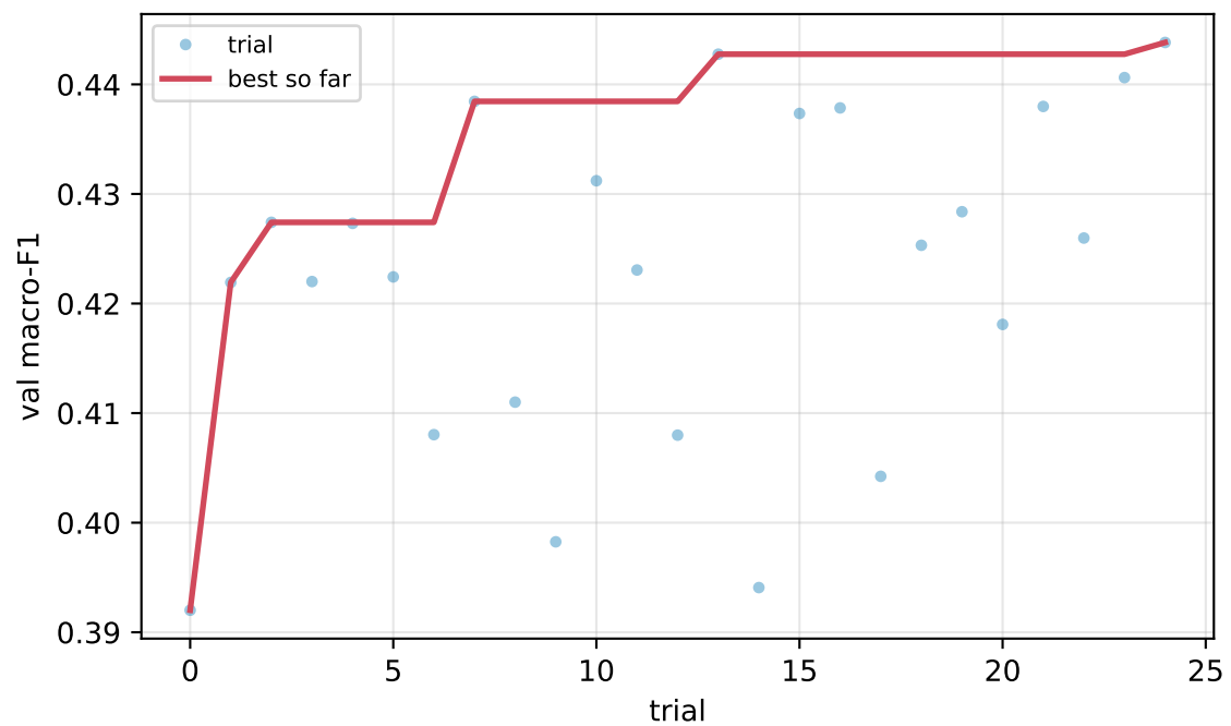
MLP
