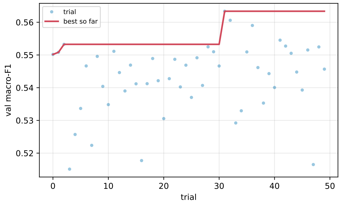
MLP
