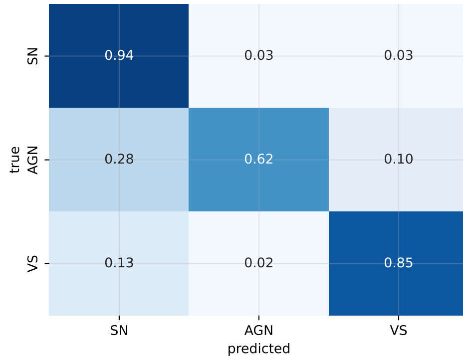
EfficientNet-B0 (F1 0.759)
