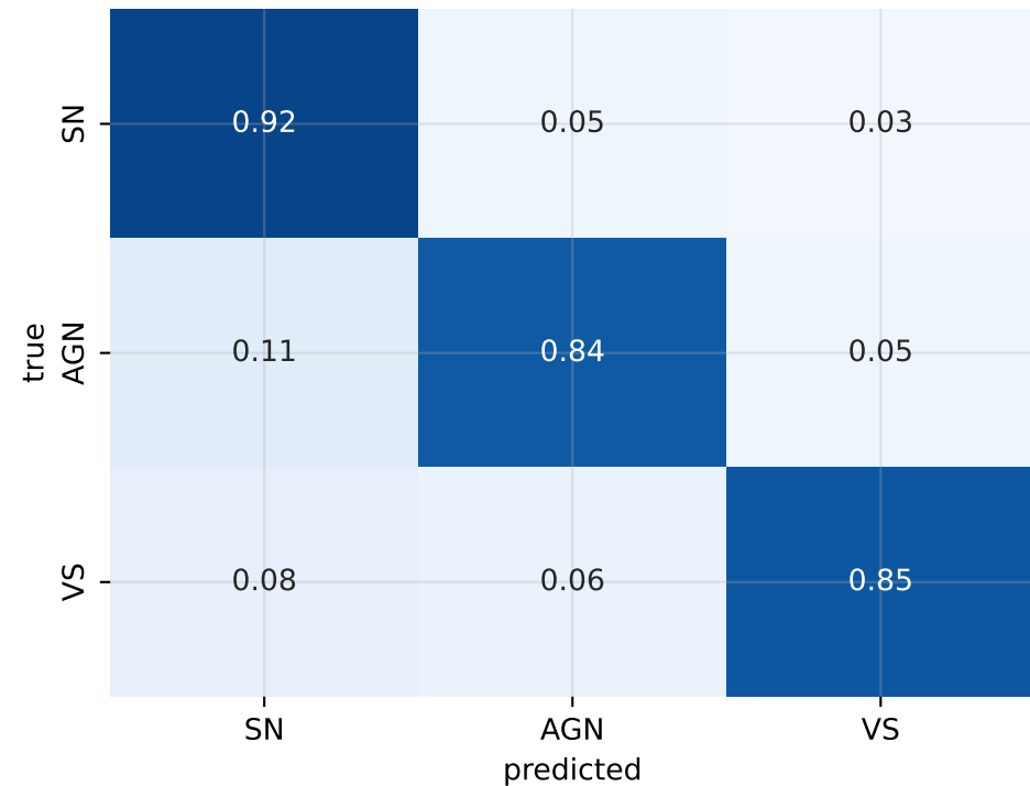
ResNet-18 (F1 0.761)
