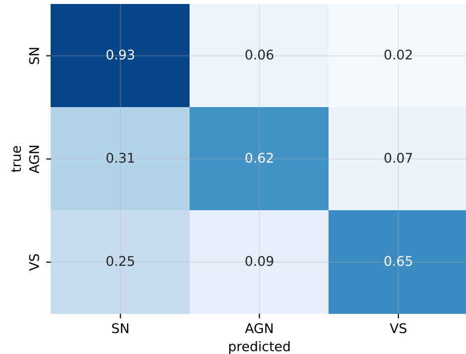
ALeRCE-CNN (F1 0.678)
