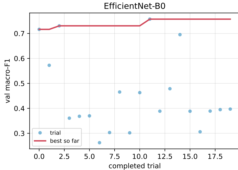
Optuna optimisation history
