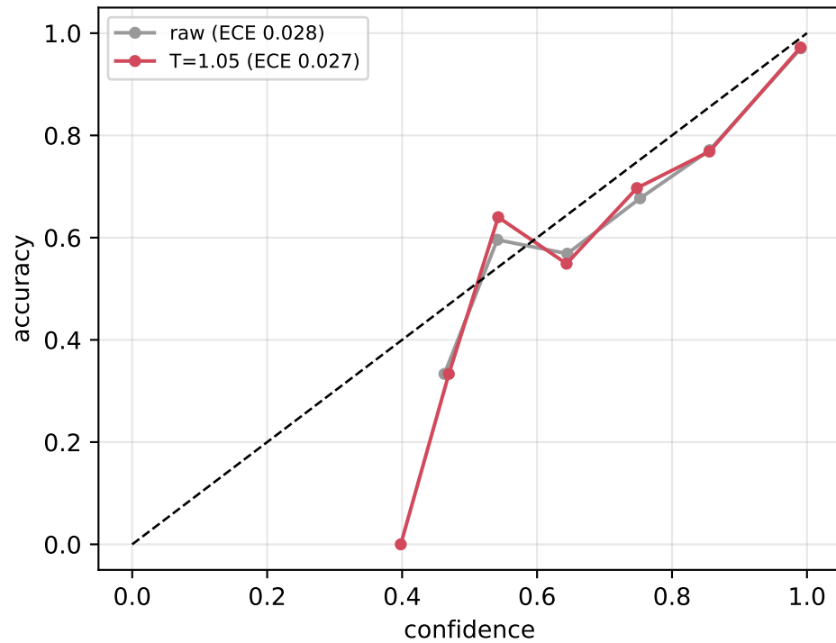
EfficientNet-B0
