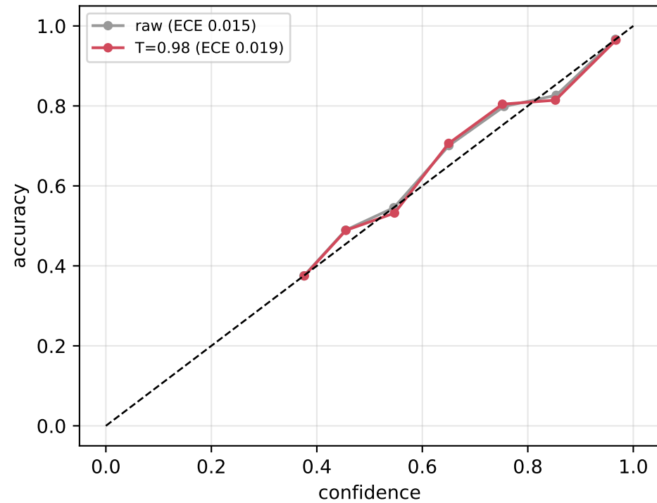
ALeRCE-CNN
