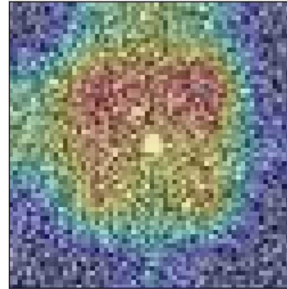
EfficientNet-B0
