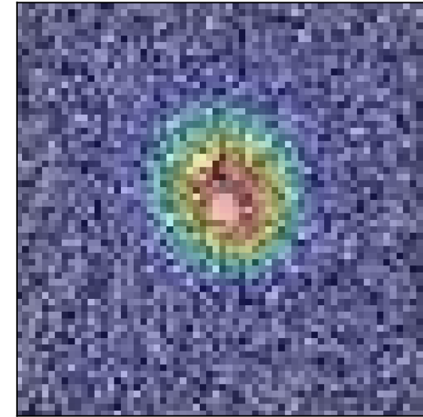
ALeRCE-CNN
