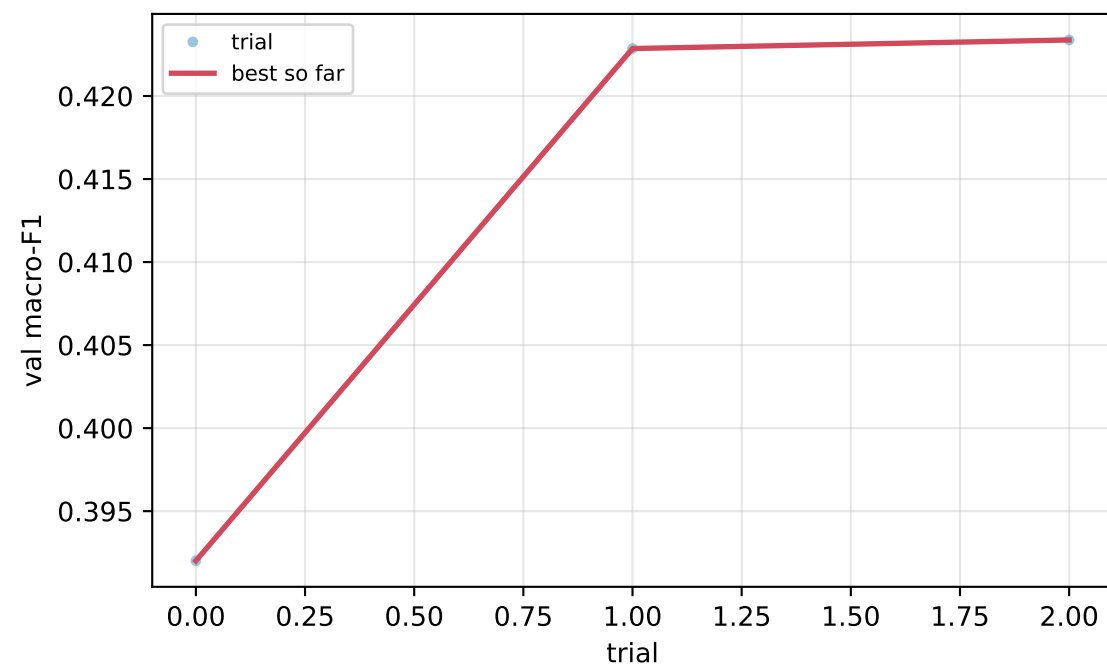
MLP
