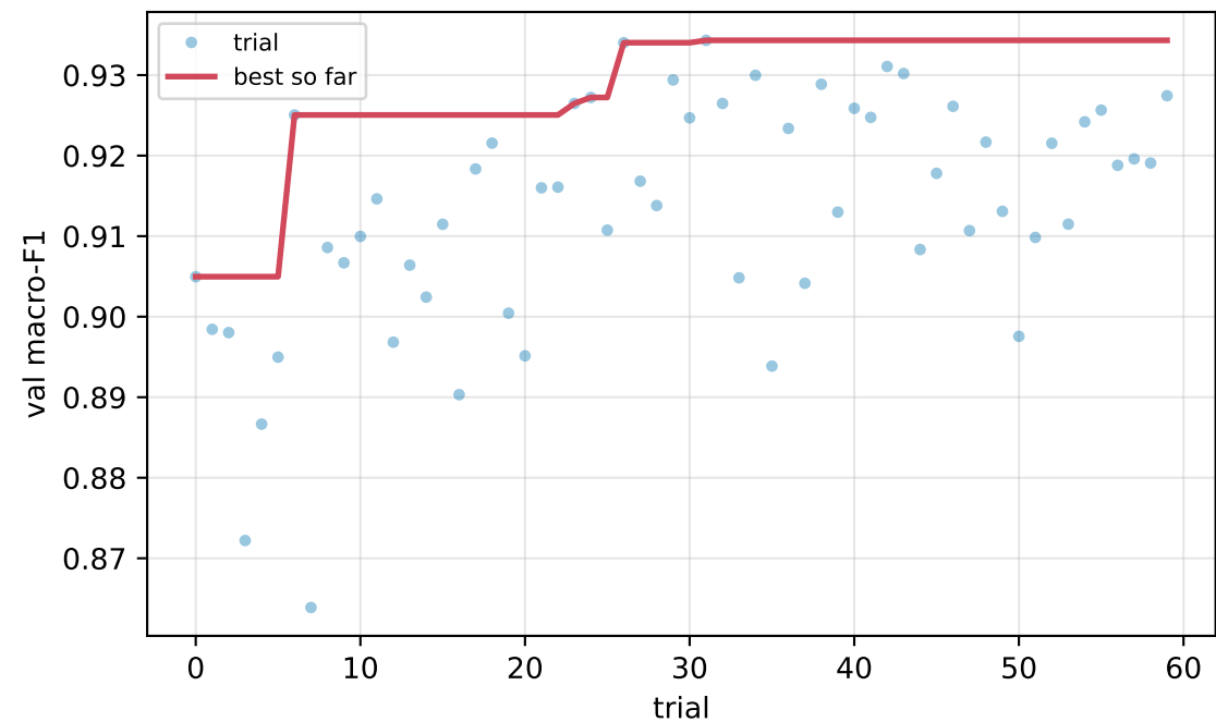
MLP
