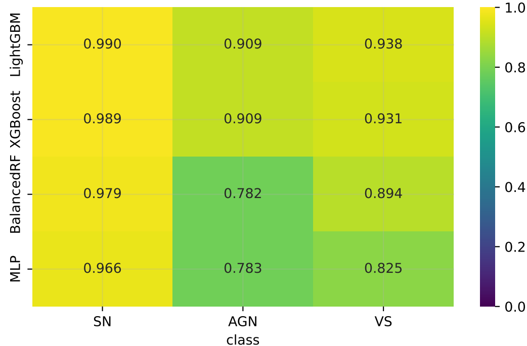
Per-class F1 — ZTF test
