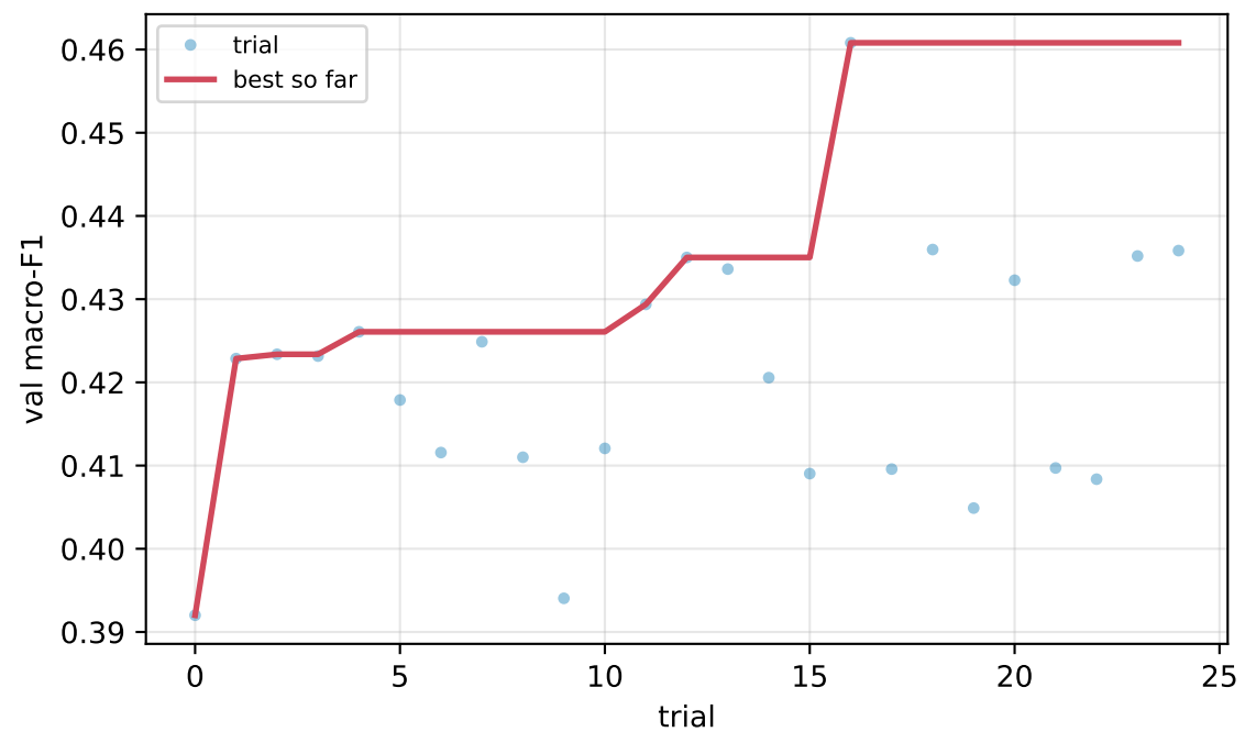
MLP
