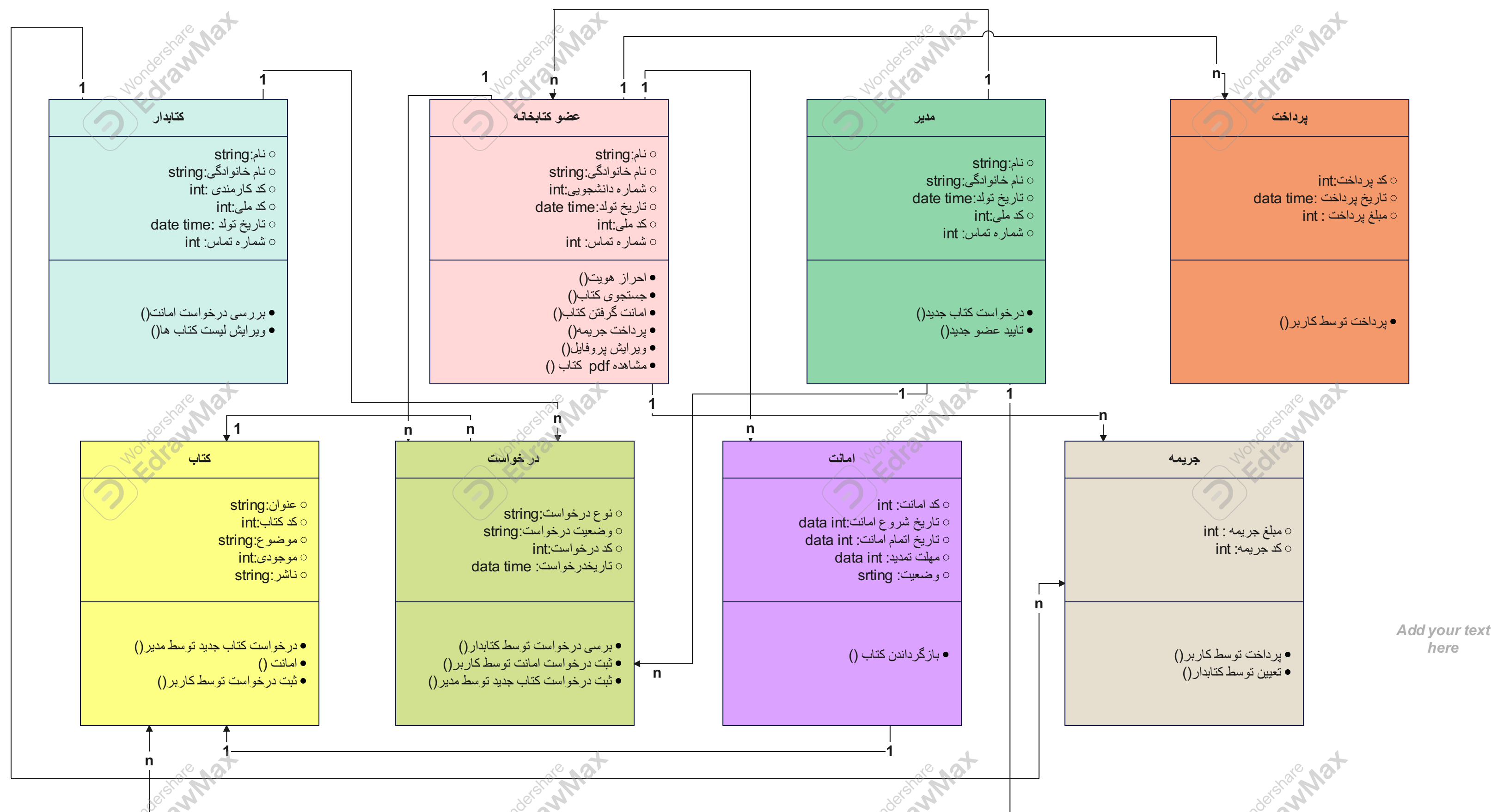
class diagram مدیریت کتابخانه
