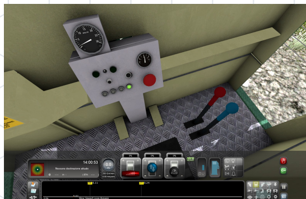
Abbildung 4 — Armaturenbrett-Detail: Motor-Drehzahlmesser (oben), Druckanzeige, roter Not-Aus-Knopf und Bedienelemente (rot/blau)
