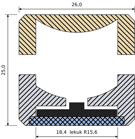
F-F x = 57,5 (dudukan pegas)
