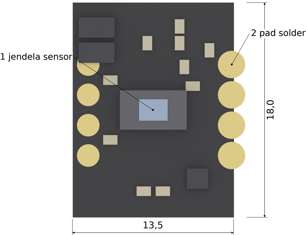
C. Tampak depan (mm)
