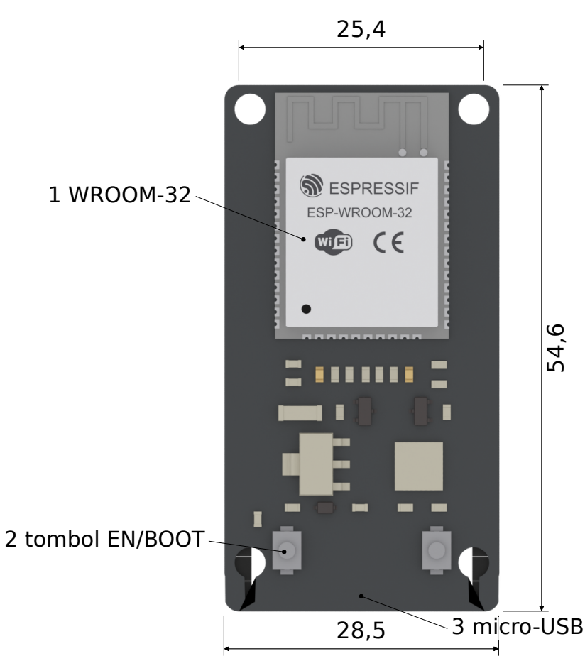
B. Tampak atas (mm)
