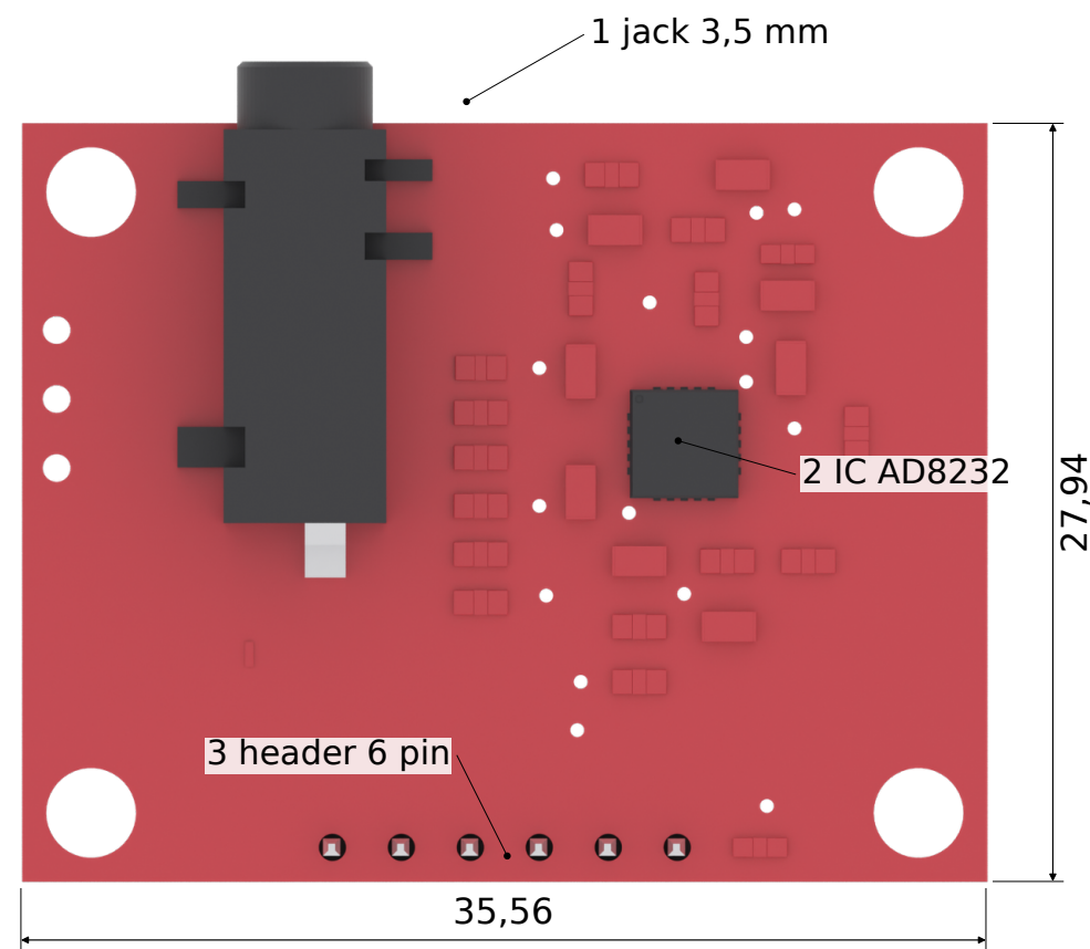
C. Tampak depan (mm)
