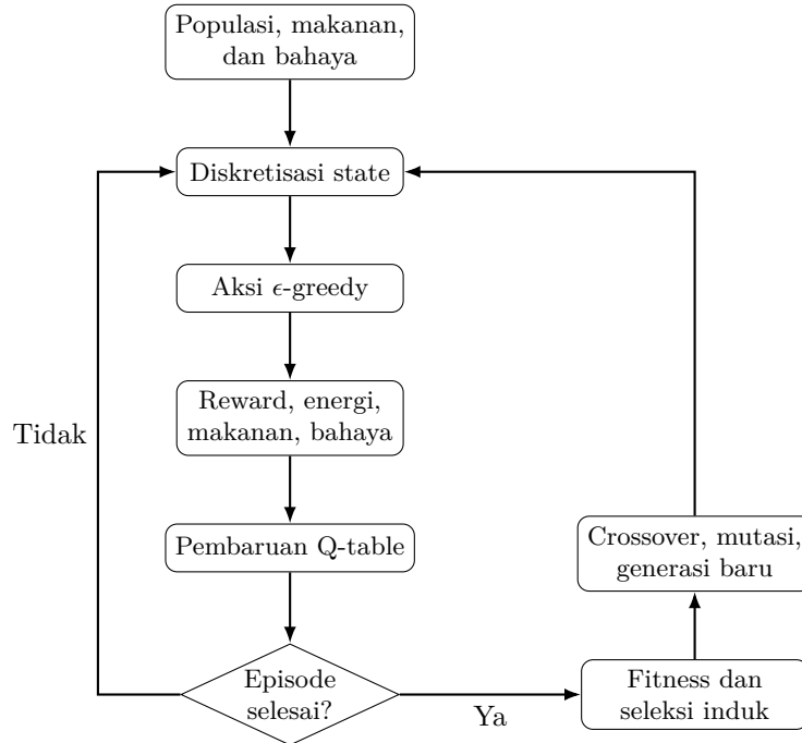
Gambar 1: Alur simulasi adaptasi agen.
