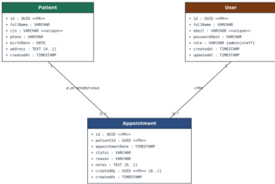
ClinicFlow — Diagramme de classes
