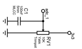
GİRİŞ-ANALOG
