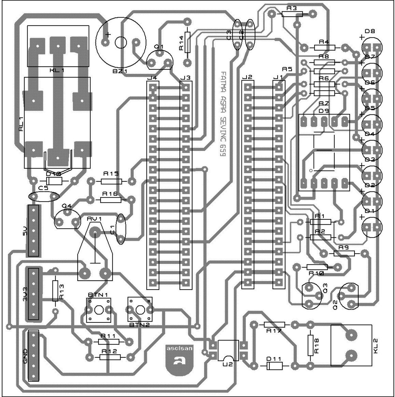
YERLEŞİM PLANI (OVERLAY)
