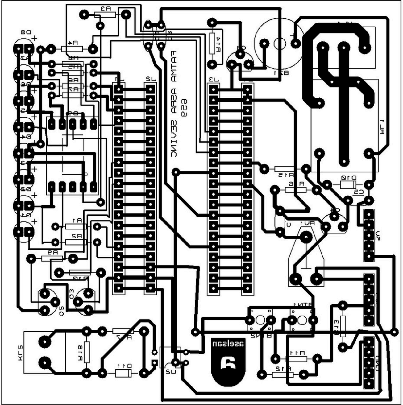
YERLEŞİM PLANI (OVERLAY)
