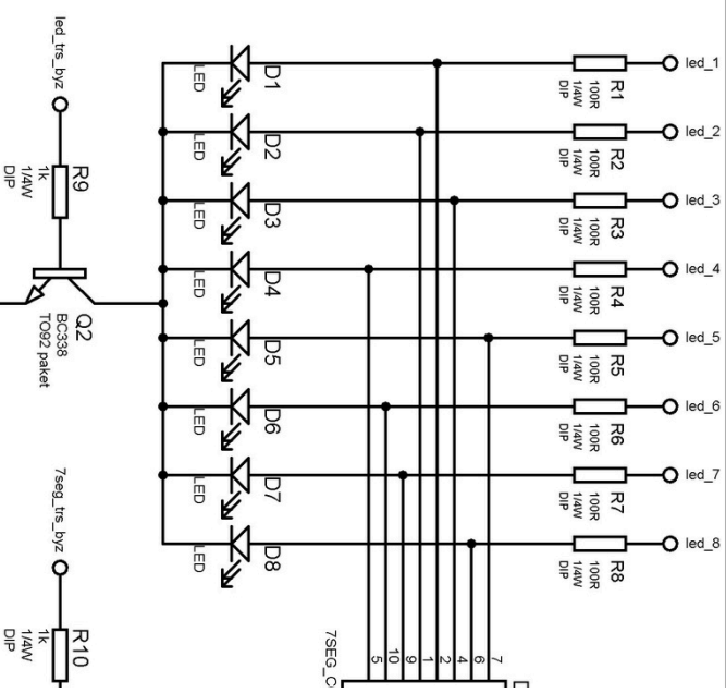
ÇIKIŞ-LED-DISPLAY
