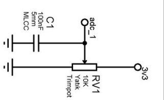
GİRİŞ-ANALOG
