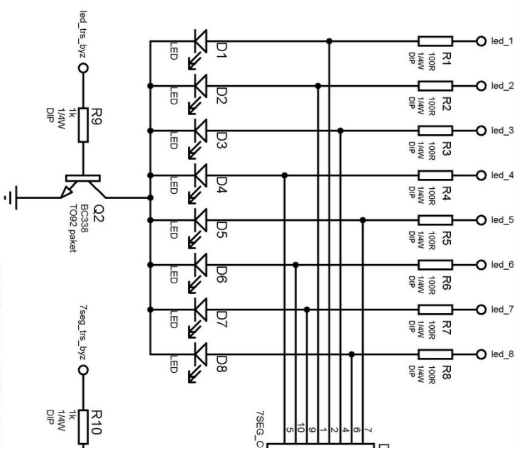
ÇIKIŞ-LED-DISPLAY
