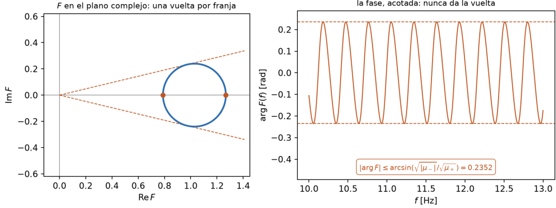
Figure 1: De dónde salen las franjas. Izquierda: el lugar geométrico de F en el plano complejo al barrer la frecuencia, una vuelta por franja. |F| queda entre el punto más cercano y el más lejano de esa circunferencia al origen, 0.7887 y 1.2679. La fase nunca da la vuelta completa, porque la circunferencia no encierra al origen: las dos tangentes desde el origen (punteadas) la acotan por \arcsin(\sqrt{|\mu_-|}/\sqrt{\mu_+}) = 0.2352 rad, que es exactamente lo que alcanza (derecha). El período de franja vale 1/\Delta T = 0.29120 Hz en cualquier punto de la banda, porque w\Delta\hat{T} es lineal en f y \Delta T es fijo — los mismos 3.434 s del eco.
