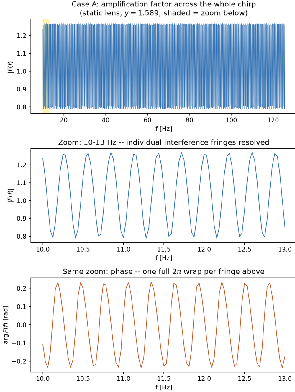
Figure 1: El factor de amplificación F(f) a través de toda la banda del chirp (arriba), con zoom a 3 Hz donde se resuelven las franjas de interferencia individuales de las dos imágenes (medio), y su fase en ese mismo zoom (abajo). w va de 62 (inicio de banda) a 778 (merger) acá — por encima de w_geo_threshold=30 , así que cada valor de F acá YA es la fórmula de óptica geométrica de dos imágenes ( theory/theory.pdf Cap. 3), no la integral de difracción exacta — confirmado reconstruyendo h_lensado a partir de nada más que dos copias retrasadas y reescaladas de la forma de onda no lensada: acuerdo con la salida real de run.py a 1.1 \times 10^{-13} , precisión de máquina. Las franjas son la interferencia entre esas dos imágenes, no un efecto de difracción adicional (ese es el régimen del Caso B, más abajo).
