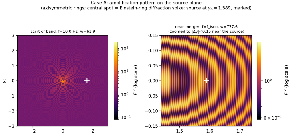
Figure 2: El patrón de amplificación extendido en el plano de la fuente: anillos de difracción concéntricos alrededor del lente con un pico brillante central de anillo de Einstein (finito en óptica de ondas, donde la magnificación de óptica geométrica diverge formalmente — el análogo en GWs de la mancha óptica de Arago/Poisson). Izquierda: patrón completo al inicio de banda ( w = 61.9 ). Derecha: zoom a |\Delta y| < 0.15 cerca del merger ( w = 777.6 ) — los mismos anillos, ahora tan cercanamente espaciados que parecen franjas casi rectas a este zoom.
