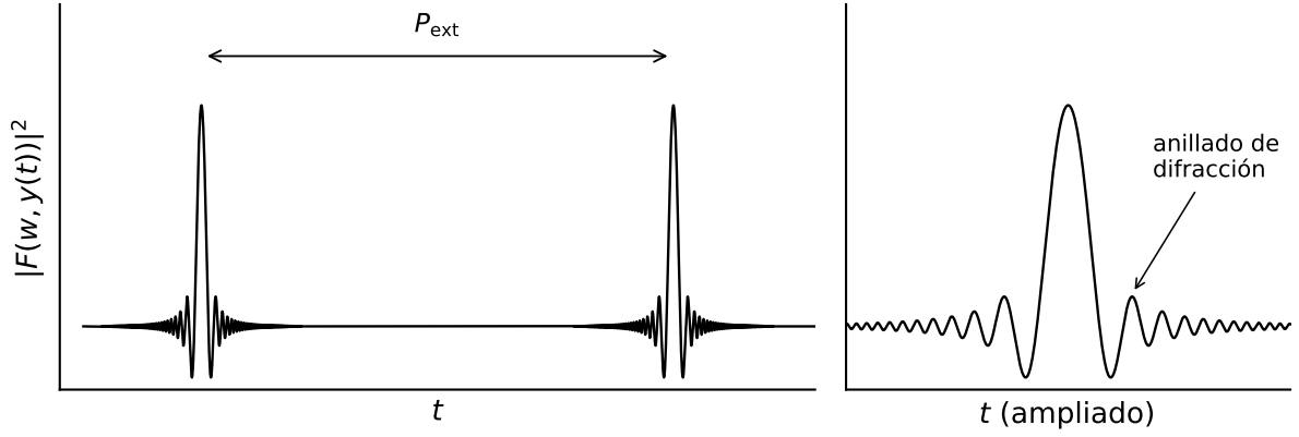
Figura 4.1: El tren de pulsos. A la izquierda, dos períodos externos: un pulso de amplificación por vuelta, y entre ellos |F|^2 = 1 , que es la mitad de órbita en la que la fuente pasa por delante del lente y no hay geometría de lente en absoluto (§4.2). A la derecha, un pulso ampliado: el anillado que lo flanquea es el patrón de difracción del capítulo 3 barrido en el tiempo, y es la firma que distingue óptica de ondas de óptica geométrica, que no lo produce. El esquema es cualitativo y no lleva números en ningún eje: la altura del pulso la fija el y mínimo de esa órbita y su ancho, la velocidad con que y barre ese mínimo.
