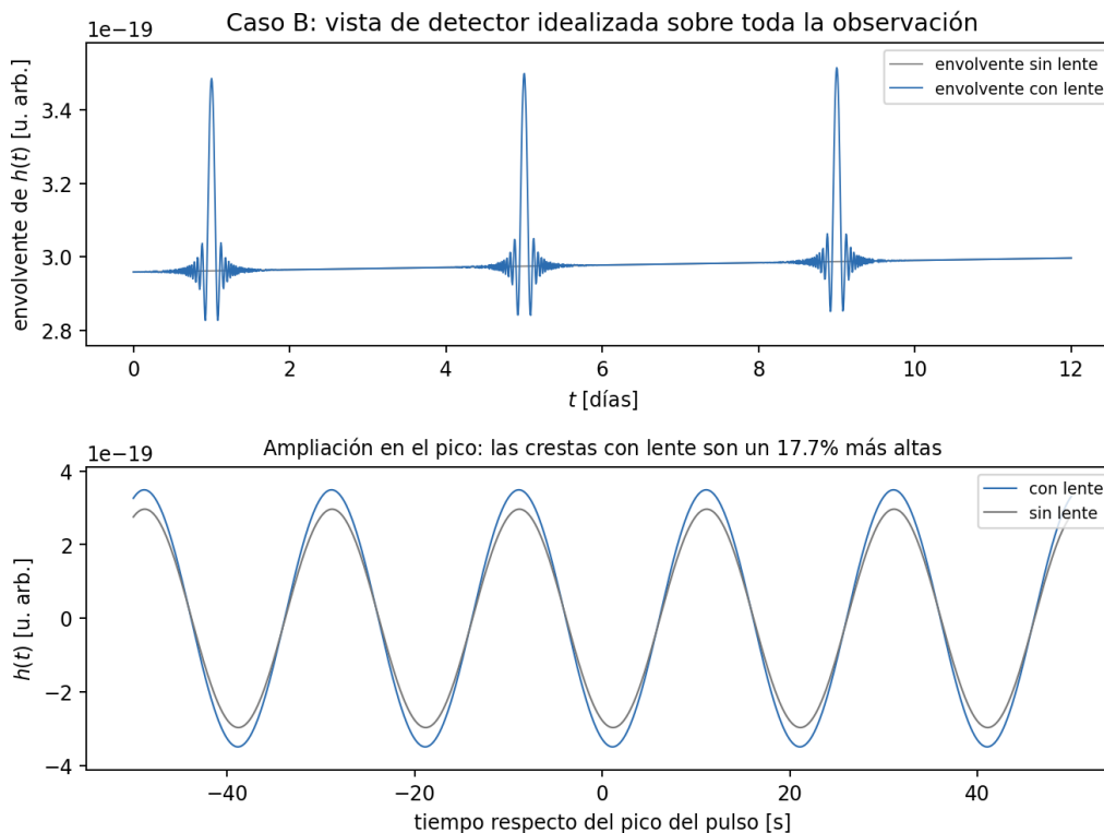
Figura 7: Vista de detector idealizada. Arriba, la envolvente de strain sobre los 12 días: tres pulsos limpios sobre una línea de base que sube un 1.29 % — esa deriva es la fuente, no el lente, y es el único lugar donde se ve que “cuasi-monocromático” no es monocromático (la binaria sigue inspirando, de 0.05000 a 0.05097 Hz, y la amplitud va como f^{2/3} ). Abajo, cinco ciclos de la portadora de 20 s en el pico de un pulso: las crestas con lente son un 17.7 % más altas. Lo que separa las dos curvas es amplitud : ambas se evalúan en el mismo tiempo retardado, así que los 90 ciclos de Roemer son comunes y se cancelan entre ellas.
