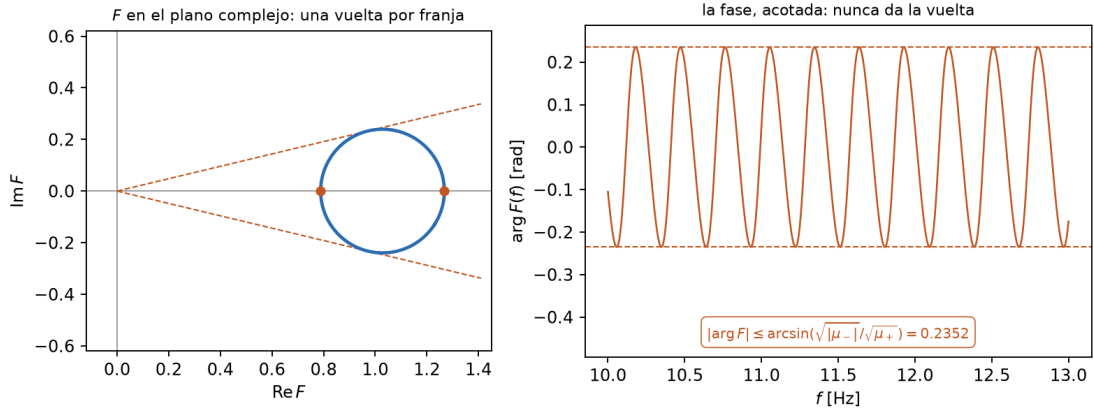
Figura 1: De dónde salen las franjas. Izquierda: el lugar geométrico de F en el plano complejo al barrer la frecuencia, una vuelta por franja. |F| queda entre el punto más cercano y el más lejano de esa circunferencia al origen, 0.7887 y 1.2679. La fase nunca da la vuelta completa, porque la circunferencia no encierra al origen: las dos tangentes desde el origen (punteadas) la acotan por \arcsin(\sqrt{|\mu_-|}/\sqrt{\mu_+}) = 0.2352 rad, que es exactamente lo que alcanza (derecha). El período de franja vale 1/\Delta T = 0.29120 Hz en cualquier punto de la banda, porque w\Delta\hat{T} es lineal en f y \Delta T es fijo — los mismos 3.434 s del eco.
