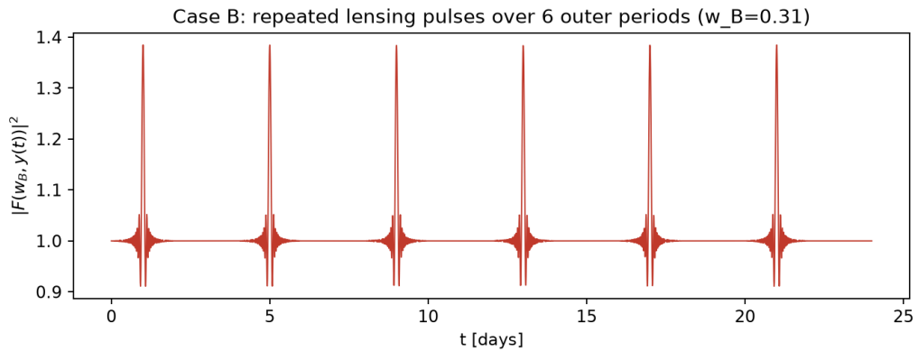
Figure 5: |F(w_B, y(t))|^2 sobre toda la observación de 24 días: seis pulsos de amplificación periódicos, uno por período externo, con pico en |F|^2 = 1.385 , con anillado (‘ringing’) de difracción visible a ambos lados de cada pico.
