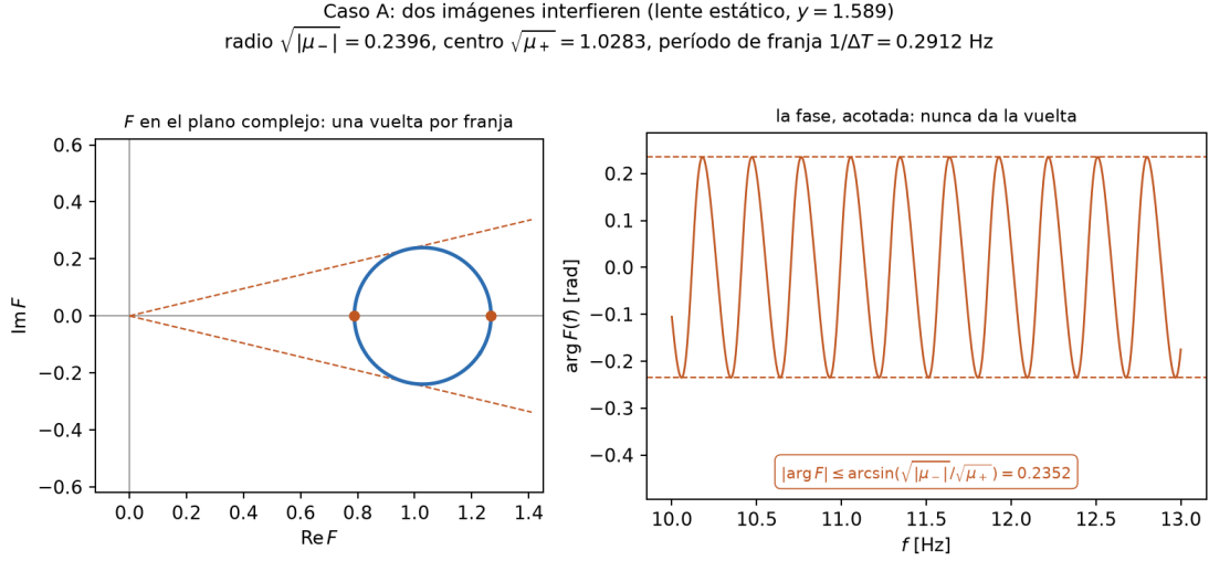
Figure 1: De dónde salen las franjas. Izquierda: el lugar geométrico de F en el plano complejo al barrer la frecuencia, una vuelta por franja. |F| queda entre el punto más cercano y el más lejano de esa circunferencia al origen, 0.7887 y 1.2679. La fase nunca da la vuelta completa, porque la circunferencia no encierra al origen: las dos tangentes desde el origen (punteadas) la acotan por \arcsin(\sqrt{|\mu_-|}/\sqrt{\mu_+}) = 0.2352 rad, que es exactamente lo que alcanza (derecha). El período de franja vale 1/\Delta T = 0.29120 Hz en cualquier punto de la banda, porque w\hat{\Delta T} es lineal en f y \Delta T es fijo — los mismos 3.434 s del eco.
