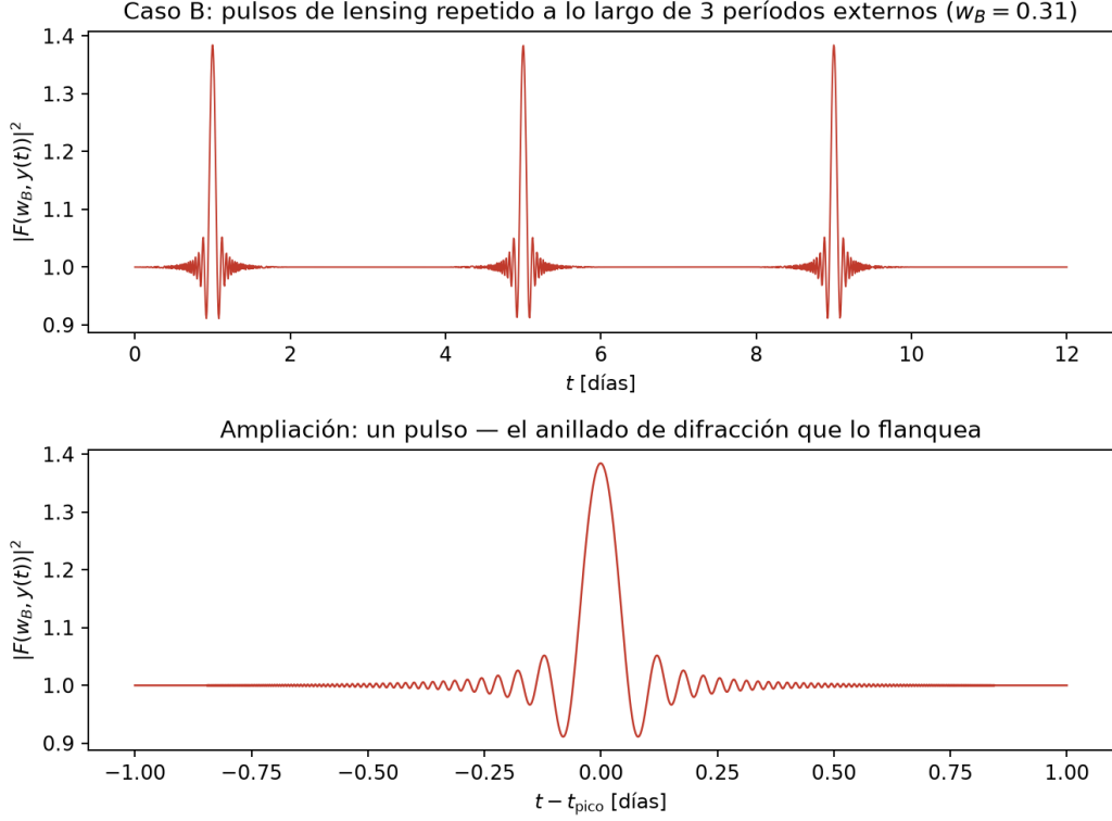
Figure 6: |F(w_B, y(t))|^2 sobre los 12 días: tres pulsos, uno por período externo, con pico en 1.3845. El panel inferior amplía uno para resolver el anillado de difracción a ambos lados, que es la firma de óptica de ondas y que la óptica geométrica no produce. Cada pulso dura unas 1.8 h a media altura, un 1.9% del período y unos 330 ciclos de portadora.
