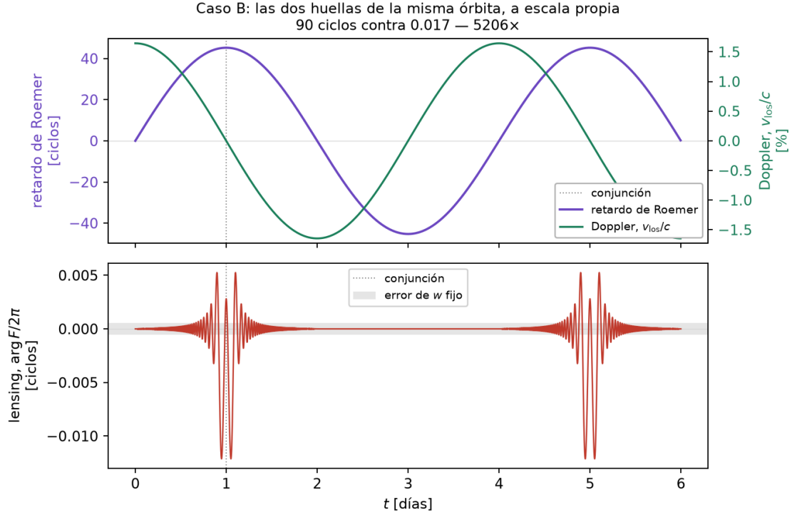
Figure 8: Las dos huellas de la misma órbita, cada una a su escala: un cociente de 5206 no se puede dibujar en un eje común. Arriba, el retardo de Roemer junto al corrimiento Doppler en eje gemelo. Abajo, la fase del lente, con el sistemático de evaluar F a w fijo dibujado como banda.
