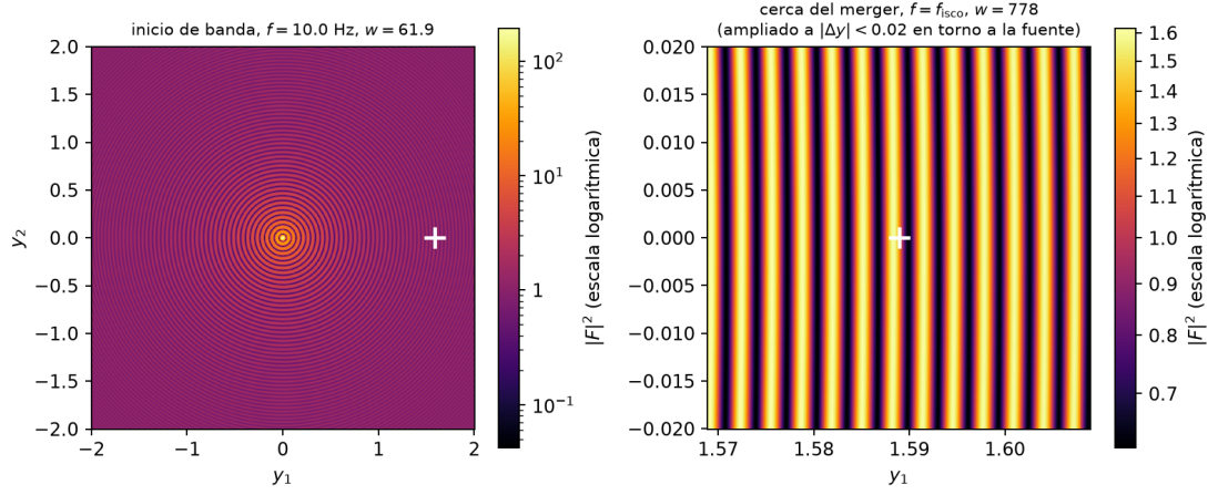
Figure 2: El patrón de amplificación en el plano de la fuente. Izquierda: patrón completo al inicio de banda ( w = 61.9 ). Derecha: ampliación a |\Delta y| < 0.02 cerca del merger ( w = 778 ) — los mismos anillos, ahora tan juntos que parecen franjas rectas. El espaciado va como 1/w , así que entre el inicio de la banda y el merger los anillos se aprietan un factor 12.5. La fuente está quieta en y_A (la cruz): lo que se mueve es la frecuencia.
