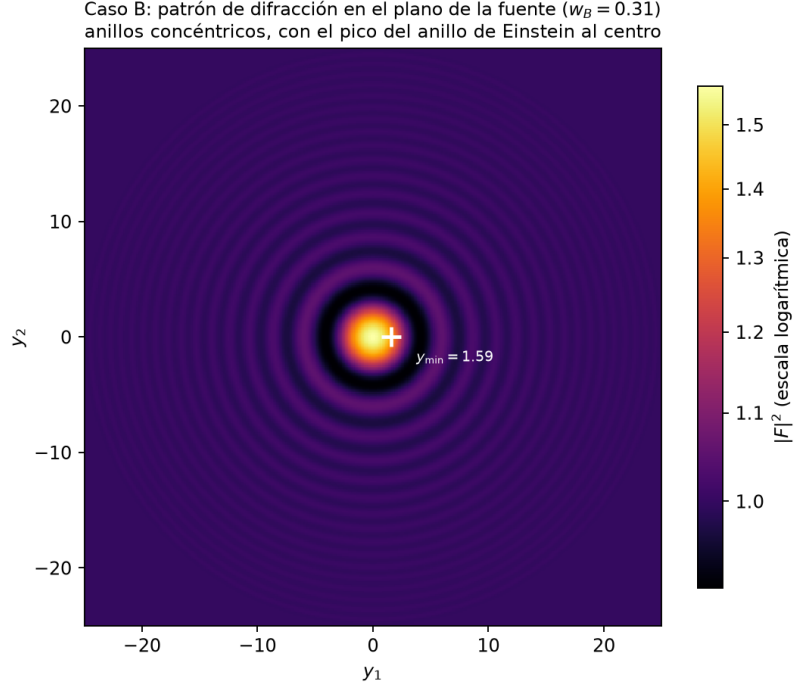
Figure 5: El patrón de difracción a w_B = 0.309 : anillos concéntricos con el pico del anillo de Einstein al centro, que en óptica de ondas es finito donde la magnificación de óptica geométrica diverge — el análogo en GWs de la mancha de Arago-Poisson. La cruz marca el acercamiento máximo de la fuente durante la observación, y_{\min} = 1.589 . Recorrer este patrón una vez por período externo es todo el Caso B.
