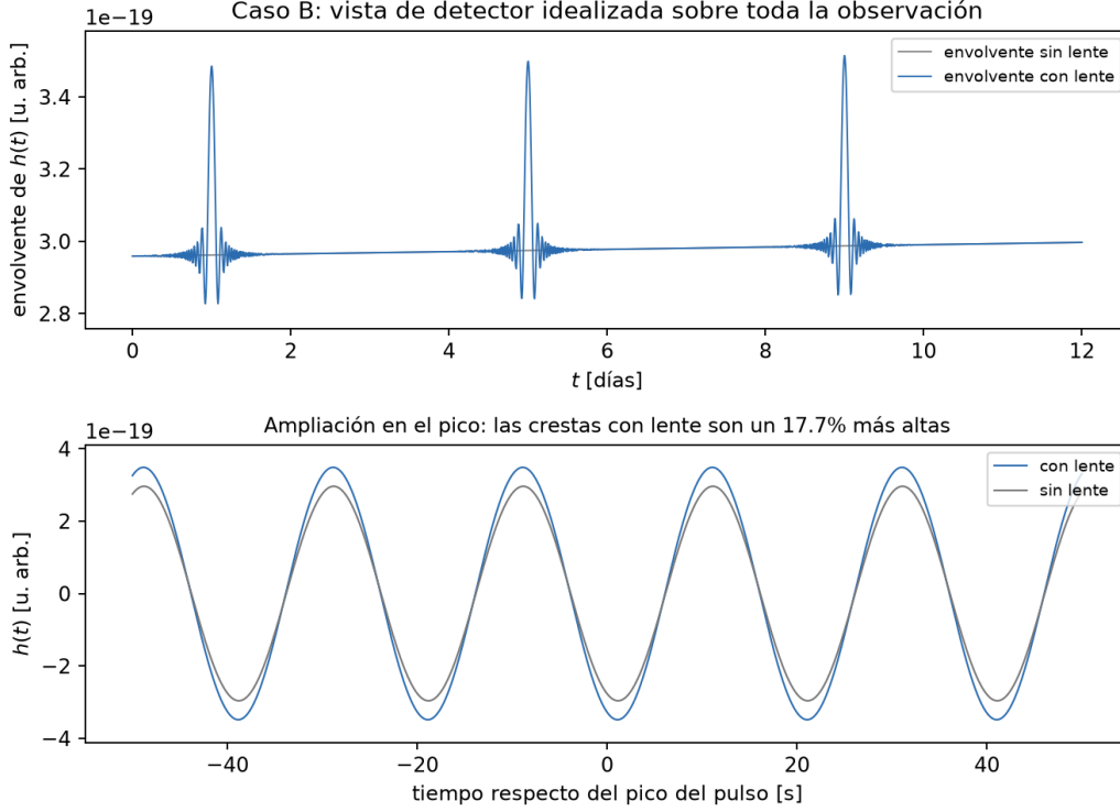
Figure 7: Vista de detector idealizada. Arriba, la envolvente de strain sobre los 12 días: tres pulsos limpios sobre una línea de base que sube un 1.29% — esa deriva es la fuente, no el lente, y es el único lugar donde se ve que “cuasi-monocromático” no es monocromático (la binaria sigue inspiralando, de 0.05000 a 0.05097 Hz, y la amplitud va como f^{2/3} ). Abajo, cinco ciclos de la portadora de 20 s en el pico de un pulso: las crestas con lente son un 17.7% más altas. Lo que separa las dos curvas es amplitud : ambas se evalúan en el mismo tiempo retardado, así que los 90 ciclos de Roemer son comunes y se cancelan entre ellas.
