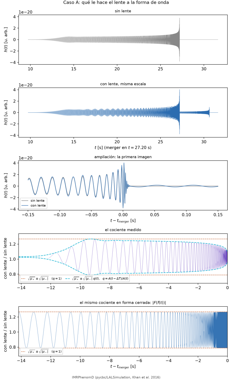
Figure 4: De arriba abajo: la señal sin lente; la misma con lente y en la misma escala, donde a simple vista no se distingue nada salvo el eco tardío; una ampliación centrada en el merger; el cociente medido de las dos envolventes, con las cotas que predice la Ec. (4) en punteado celeste; y ese mismo cociente en forma cerrada, |F(f(t))| , que es el límite q = 1 .
