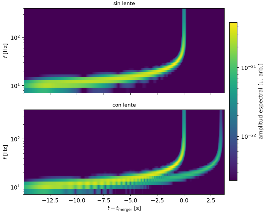
Figure 3: El chirp en tiempo-frecuencia. Arriba sin lente: una traza que barre hacia arriba hasta el merger. Abajo con lente: dos , la misma traza repetida \Delta T = 3.43 s más tarde y a \sqrt{|\mu_-|} = 0.24 de la amplitud. Dos imágenes son dos trazas — toda la óptica geométrica del lensing en una figura. El moteado a lo largo de la traza lensada a baja frecuencia es la interferencia entre ambas.
