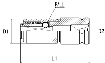
BH-3, BH-4A
