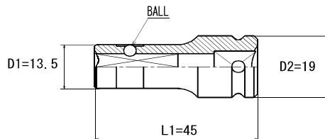
BH-38
