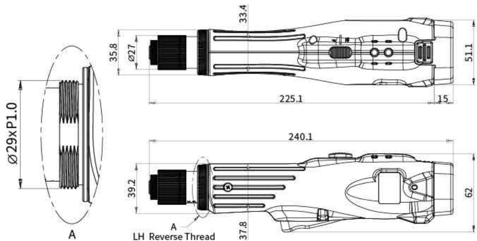
MYBT-AS0212 Unit: mm
