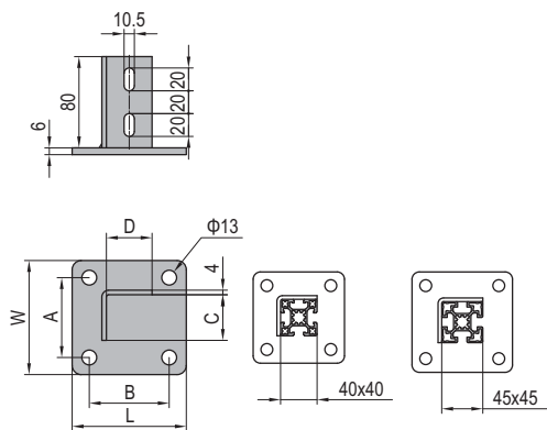
Base Plate 40x40/45x45 隔断支脚 40x40/45x45
