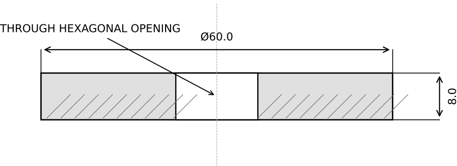
(c) SECTION A--A
