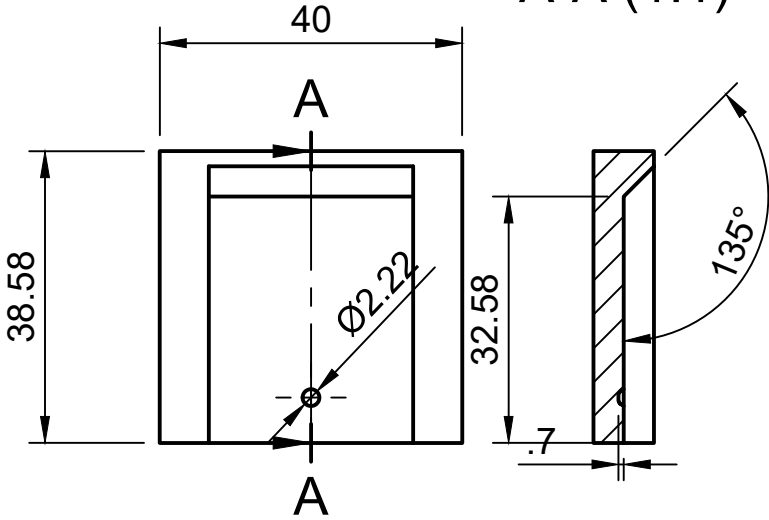
A-A (1:1)
