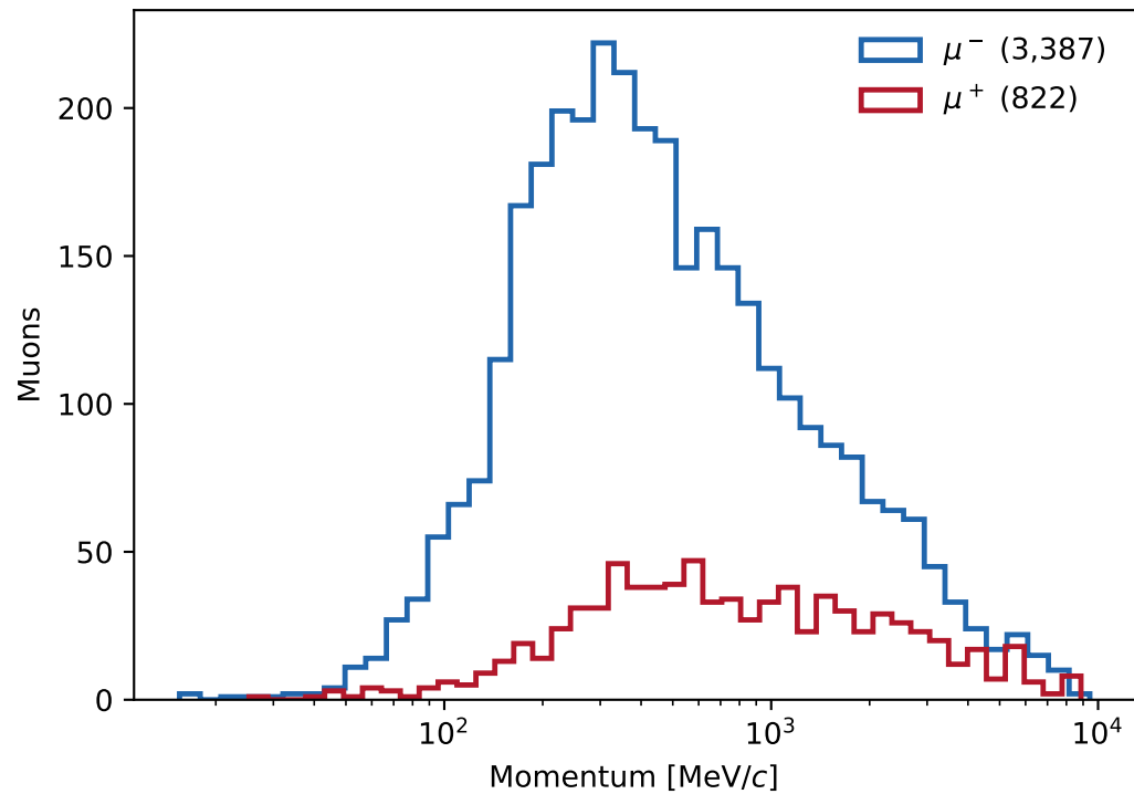
Muon momentum
