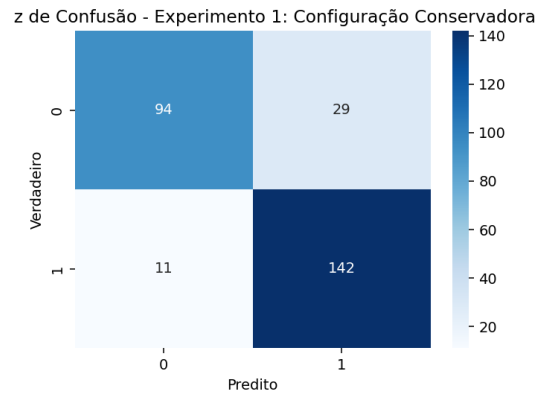
Matriz de Confusão
