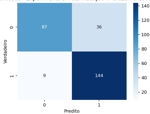
Matriz de Confusão
