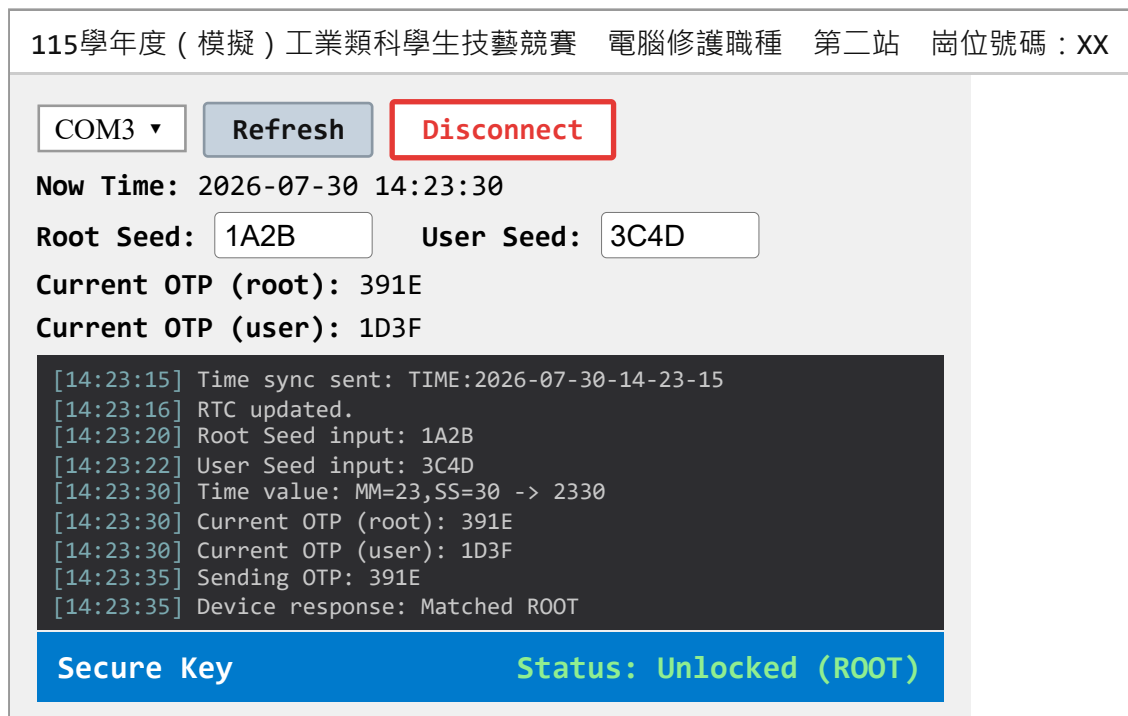
圖 6 電腦執行視窗畫面（參考用，含 Seed 欄位、OTP 即時值與完整通訊交握日誌）
