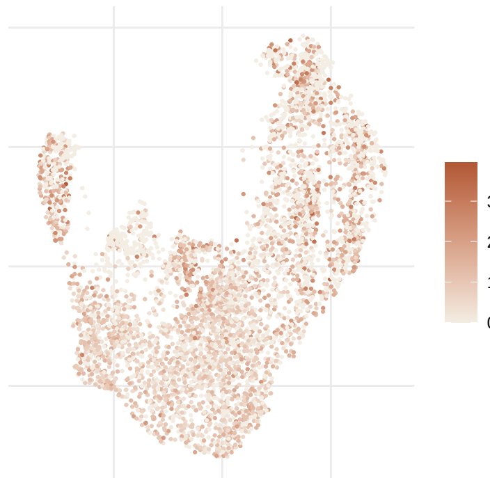
BATF3
