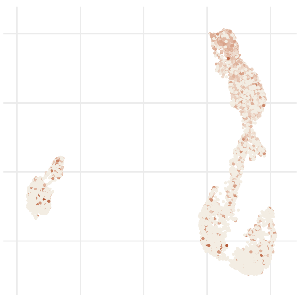
XBP1
