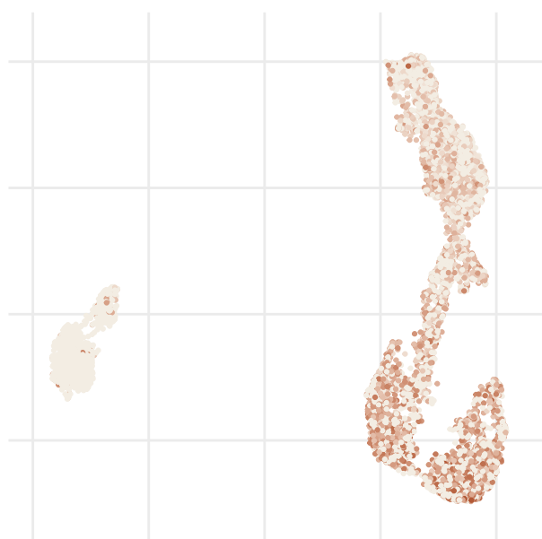
PRDM1
