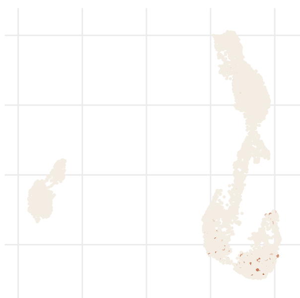
SDC1
