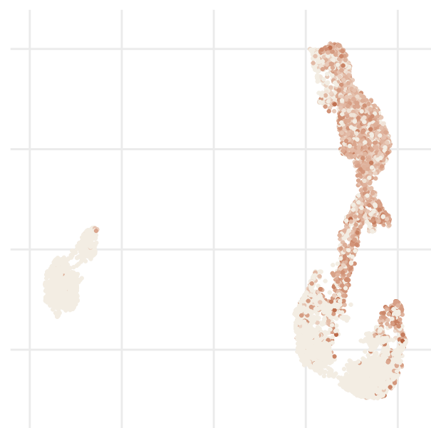
IRF4
